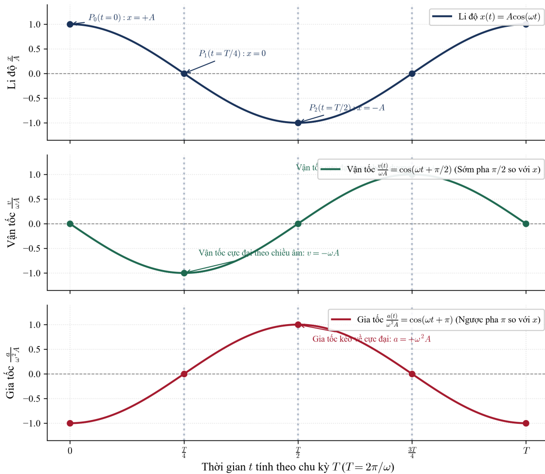
Hình 4: Hình 1.1: Đồ thị động học chuẩn hóa theo thời gian của dao động điều hòa: Li độ x(t) (xanh navy), Vận tốc v(t) (xanh lá), và Gia tốc a(t) (đỏ thẫm) qua 4 mốc thời gian kinh điển 0, T/4, T/2, 3T/4 .
