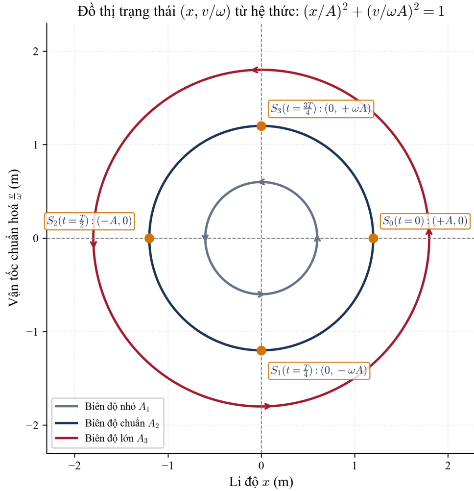
Hình 5: Hình 1.2: Đồ thị không gian trạng thái (x, v/\omega) . Quỹ đạo của dao động điều hòa là một đường tròn bán kính A quay thuận chiều kim đồng hồ, quét qua 4 mốc động học S_0, S_1, S_2, S_3 .
