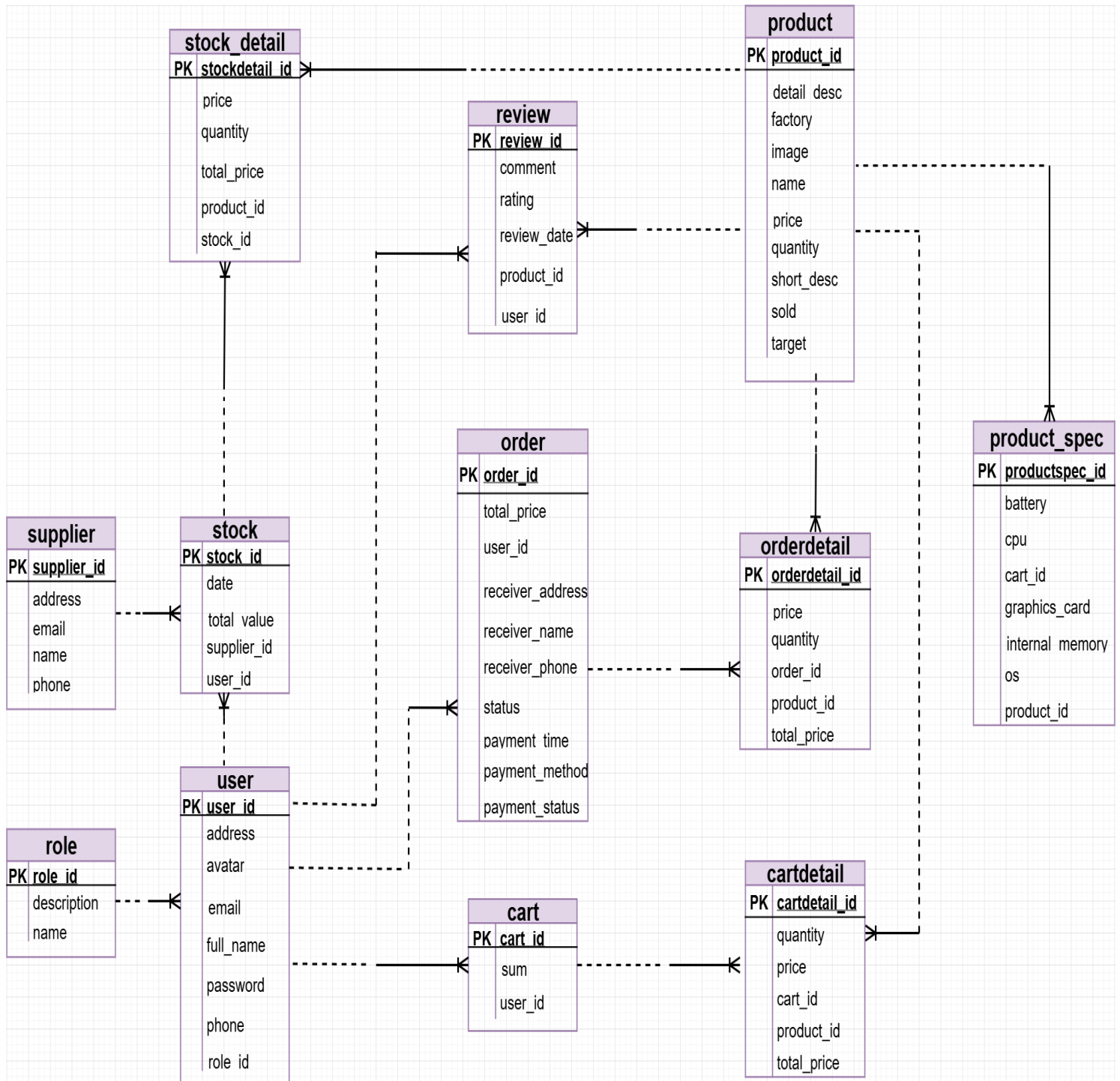
Hình 2.2. Sơ đồ quan hệ thực thể ERD hệ thống
