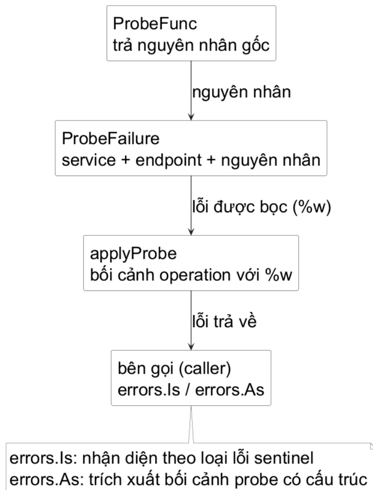
Hình 17 — Biên lỗi không nuốt nguyên nhân. Mỗi lớp chỉ thêm context mà nó thực sự biết; bên gọi chọn errors.Is khi cần một quyết định theo loại lỗi và errors.As khi cần dữ liệu từ một error cụ thể.
