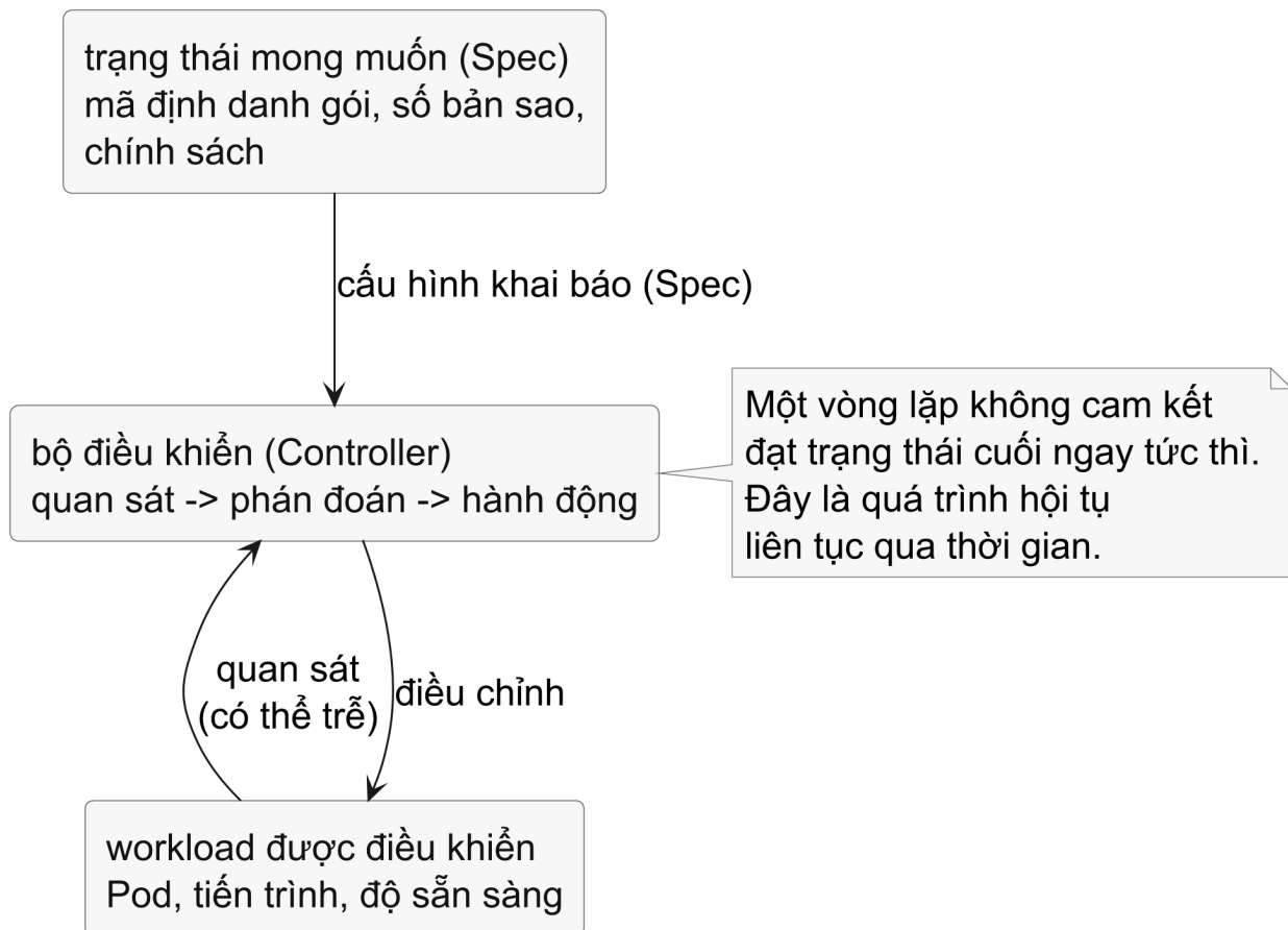
Hình 27 — Desired state là input bền hơn một lệnh start. Controller chạy nhiều vòng; trạng thái cluster có thể luôn thay đổi.
