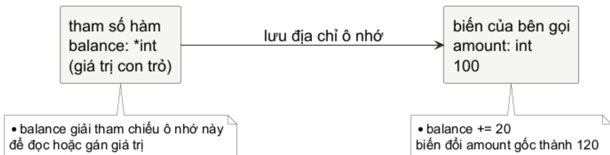
Hình 12 — balance trong function là pointer value được truyền theo value. *balance truy cập pointee; số đồ cổ ý không dùng địa chỉ số hay stack/heap để tránh biến mental model thành chi tiết runtime.
