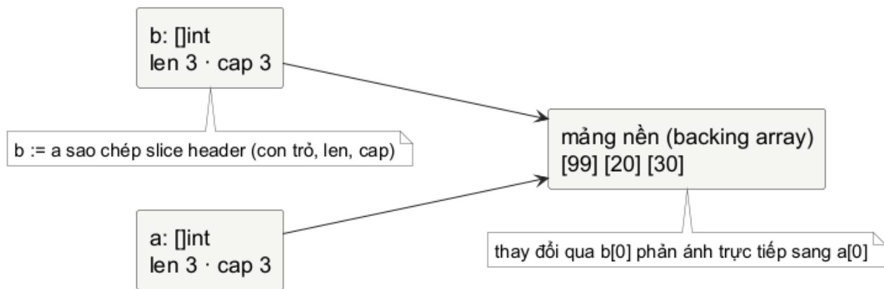
Hình 8 — b := a sao chép slice value, gồm của sổ nhìn vào dữ liệu, len và cap. Cả hai descriptor vẫn dẫn tới cùng underlying array, nên b[0] thay đổi phần tử mà a cũng nhìn thấy.
