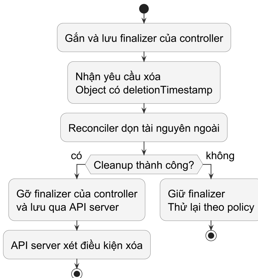
Hình 40 — Cleanup thất bại giữ finalizer để có thể thử lại. Cleanup thành công chỉ cho phép gỡ finalizer của controller này; API server còn phải xét các điều kiện xóa khác.
