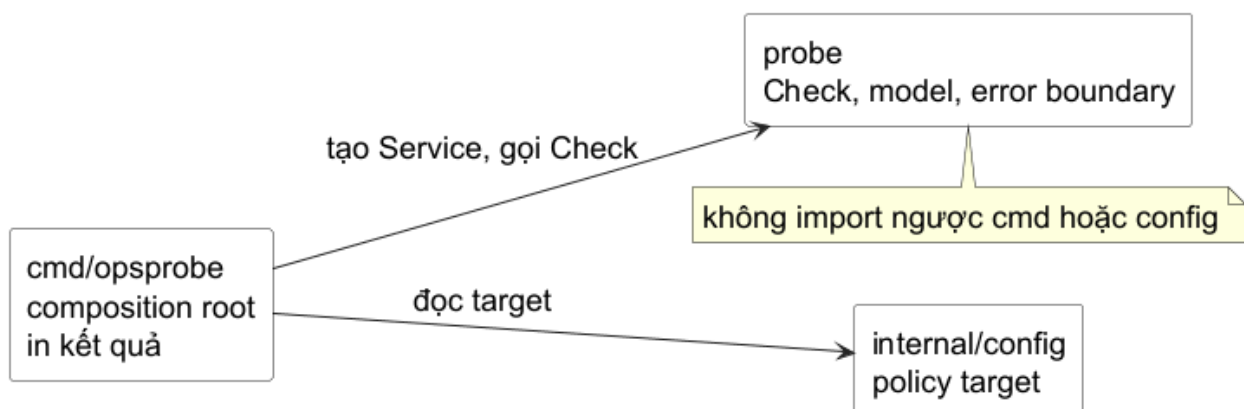
Hình 18 — Dependency direction là công cụ review. cmd/opsprobe là composition root ; nó biết các package cụ thể. probe không biết CLI hay config source nên có thể được đọc, test và thay thế runner mà không kéo presentation theo.
