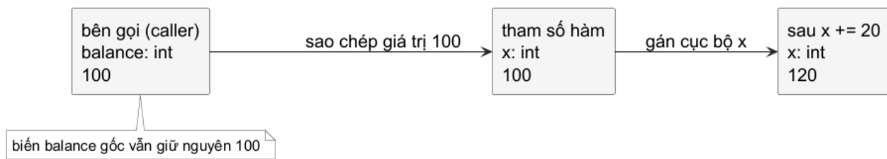
Hình 11 — Lỗi gọi addBonus(balance) copy value 100 vào parameter x . Sơ đồ biểu diễn semantics của variable và value, không khẳng định vị trí vật lý của chúng trong RAM.
