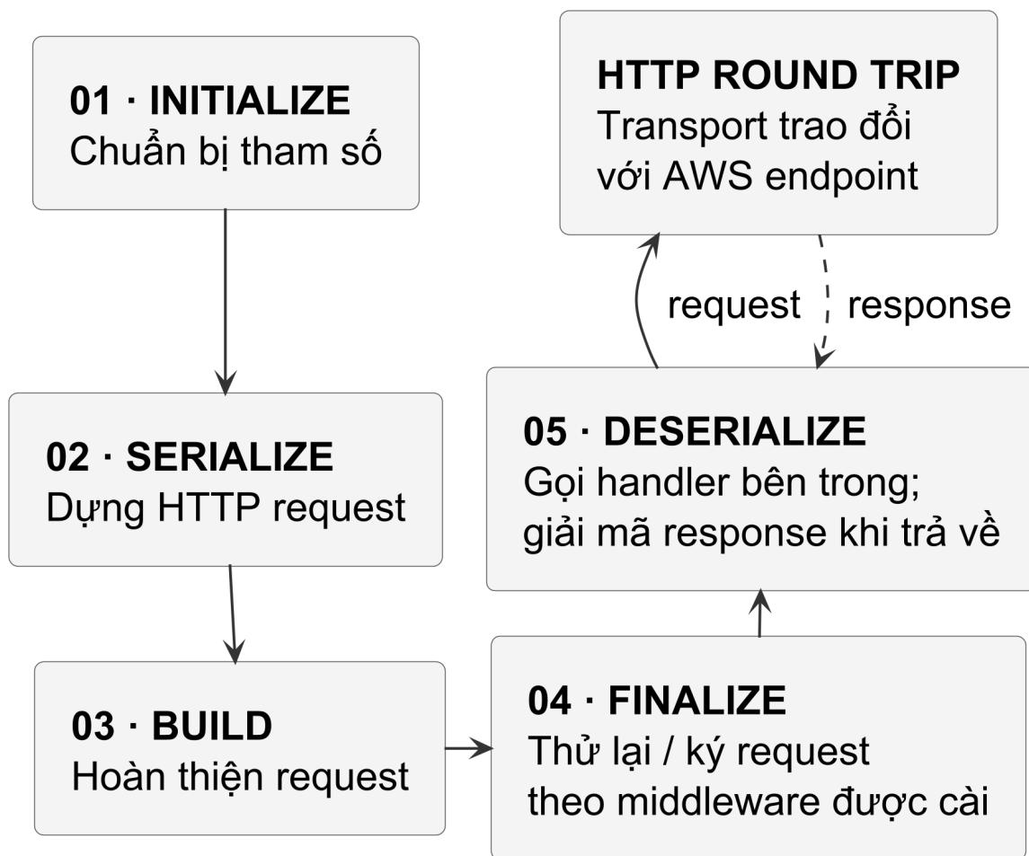
Hình 42 — Mũi tên liền biểu diễn đường gọi vào handler, mũi tên đứt biểu diễn response trở về Deserialize. Middleware cụ thể và vị trí xử lý checksum phụ thuộc operation cùng cấu hình; sơ đồ không mô tả từng lần retry.
