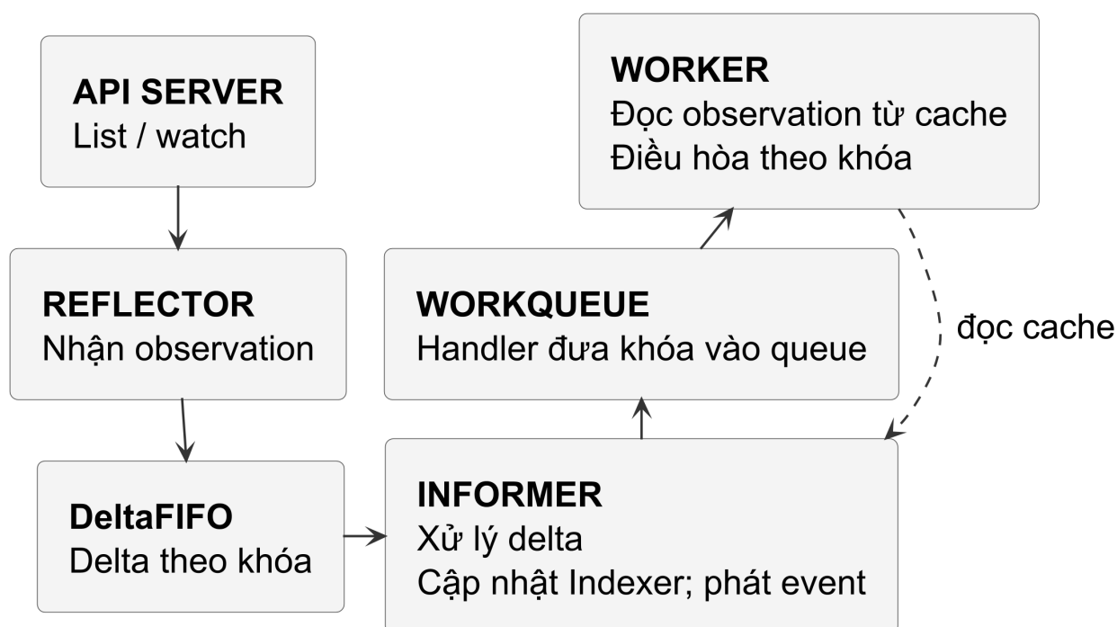
Hình 51 — Informer cập nhật cache rồi phát event tới handler; handler của ứng dụng đưa khóa vào workqueue. Worker đọc observation hiện có khi điều hòa, không coi payload event là trạng thái cuối cùng.
