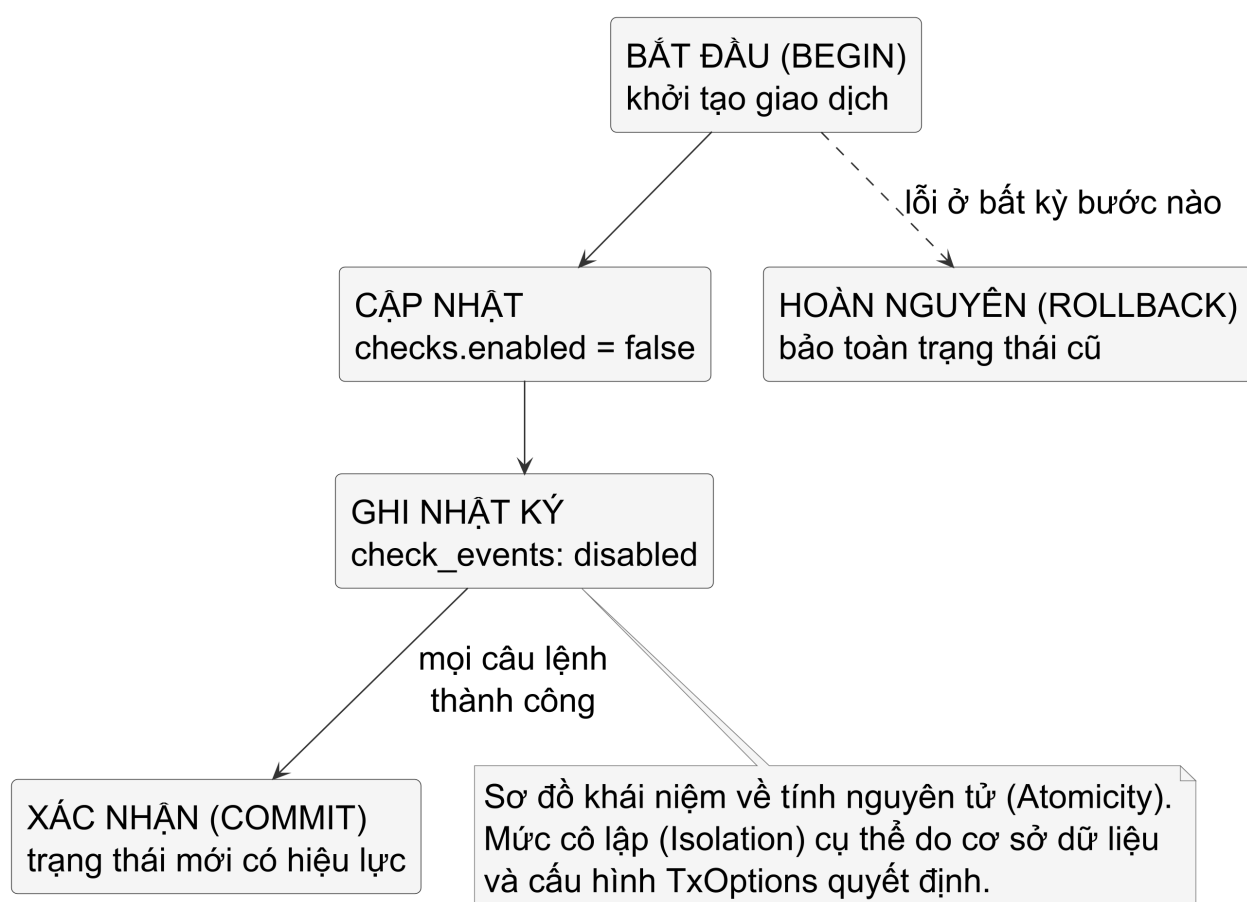
Hình 25 — Sơ đồ khái niệm về atomicity của thao tác Disable . Hình không khẳng định isolation level nào; database, driver và TxOptions mới quyết định chi tiết isolation hỗ trợ được.
