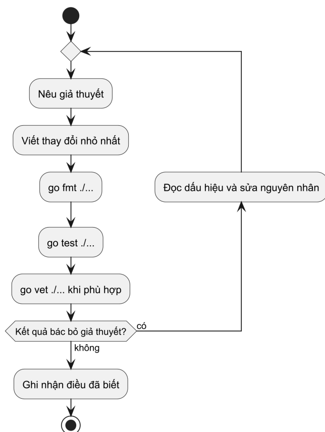
Hình 3 — Vòng lặp phản hồi giả thuyết - đo đạc - sửa mã nguồn. Trình biên dịch không phải là chướng ngại vật; trình biên dịch là công cụ kiểm định tính sớm nhất cho các dự đoán của bạn.
