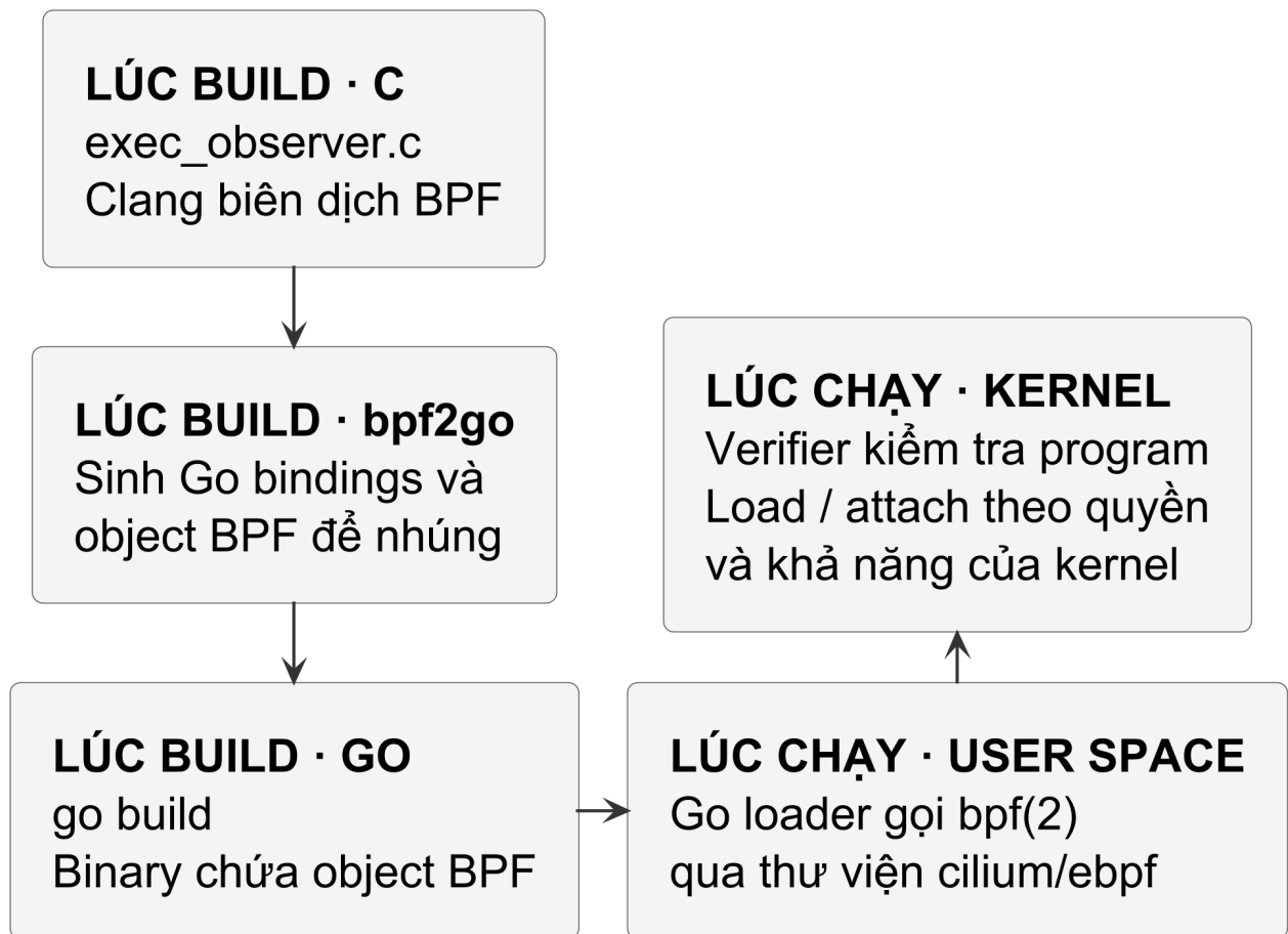
Hình 49 — Clang và bpf2go thuộc toolchain build. Binary Go mang object BPF đến runtime; kernel vẫn kiểm tra program, quyền và khả năng hỗ trợ trước khi load hoặc attach thành công.
