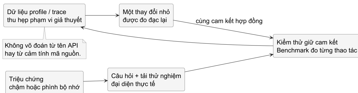
Hình 22 — Chu trình điều tra hiệu năng hoàn chỉnh. Dữ liệu bắt đầu từ một bài toán đo lường có khối lượng công việc đại diện, kiểm chứng qua profiler, sau đó đối chiếu mã nguồn và tối ưu hóa có đo đạc đối chứng.
