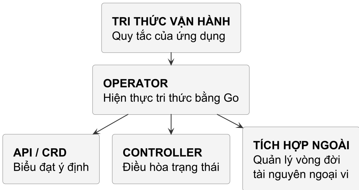
Hình 38 — Operator biểu đạt tri thức vận hành qua API, vòng lặp điều hòa và các tích hợp quản lý tài nguyên. Các thành phần này là vai trò thiết kế, không phải ba bước chạy tuần tự.
