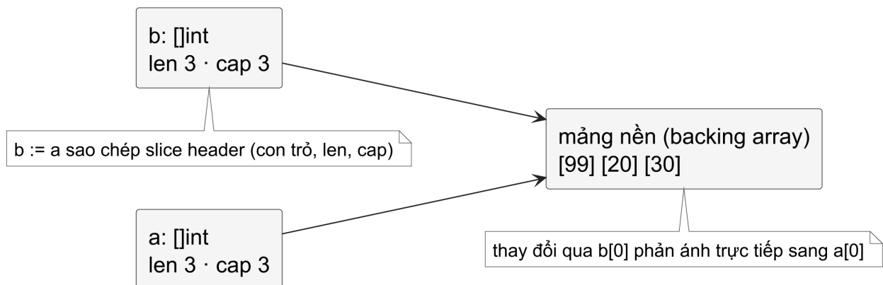
Hình 8 — b := a copy slice value, gồm cửa sổ nhìn vào dữ liệu, len và cap . Cả hai descriptor vẫn dẫn tới cùng underlying array, nên b[0] thay đổi phần tử mà a cũng nhìn thấy.
