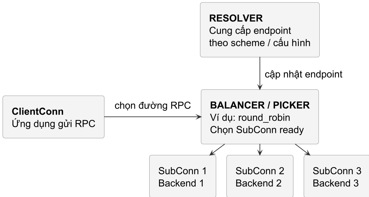
Hình 55 — Resolver cung cấp endpoint, balancer quản lý SubConn và picker chọn đường cho RPC. Ba backend cùng policy round_robin là cấu hình minh họa, không phải mặc định của mọi ClientConn.
