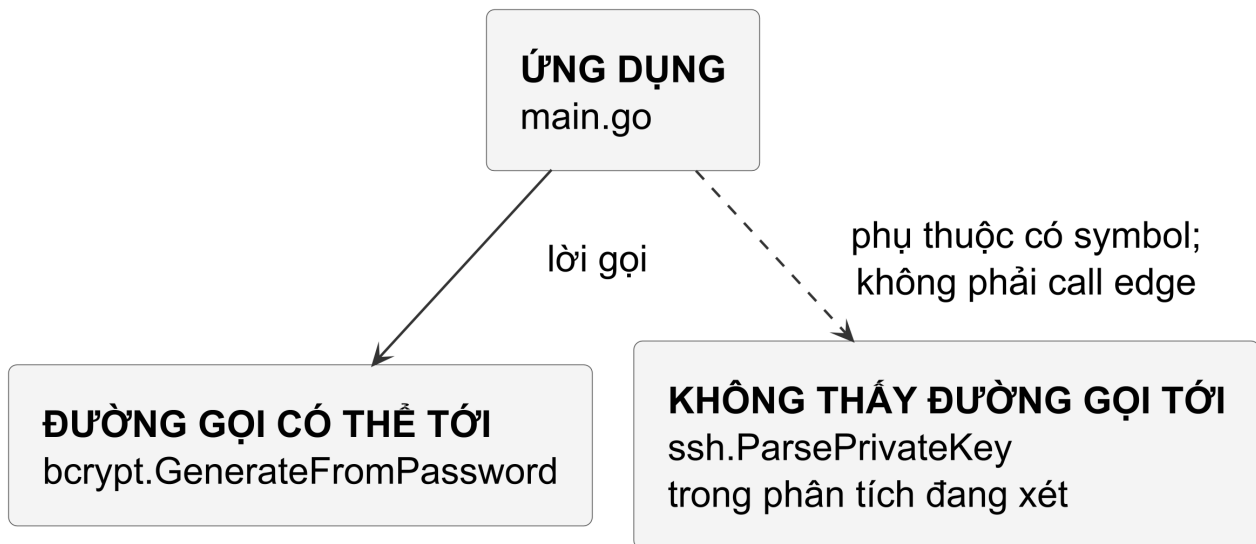
Hình 47 — Trong ví dụ phân tích này, ứng dụng có đường gọi tới bcrypt nhưng không thấy đường gọi tới ssh.ParsePrivateKey . Kết quả phải được hiểu trong giới hạn của bộ phân tích và build đang xét.
