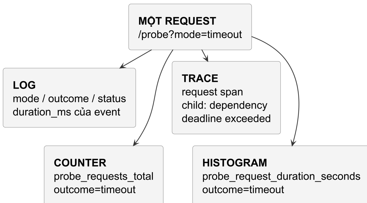
Hình 28 — Cùng request cung cấp dữ liệu cho log, trace, counter và histogram. Các đường ghi nhận thể hiện những góc nhìn khác nhau, không phải log sinh counter hay trace sinh histogram.
