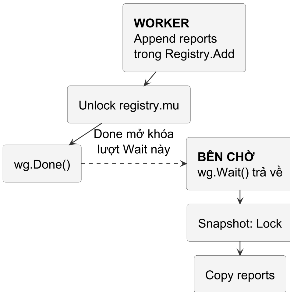
Hình 20 — Đường chứng minh cho một worker: các bước trong từng goroutine giữ thứ tự code; cạnh đứt là quan hệ Done mở khóa lượt Wait này. Snapshot chỉ chạy sau khi Wait trả về.
