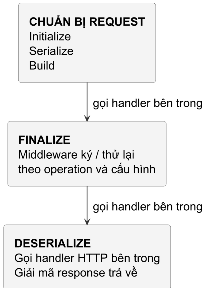
Hình 52 — Năm step tổ chức đường gọi vào bên trong. Deserialize gọi handler HTTP trước khi giải mã response; sơ đồ lược bỏ đường response đi ngược ra ngoài các step.
