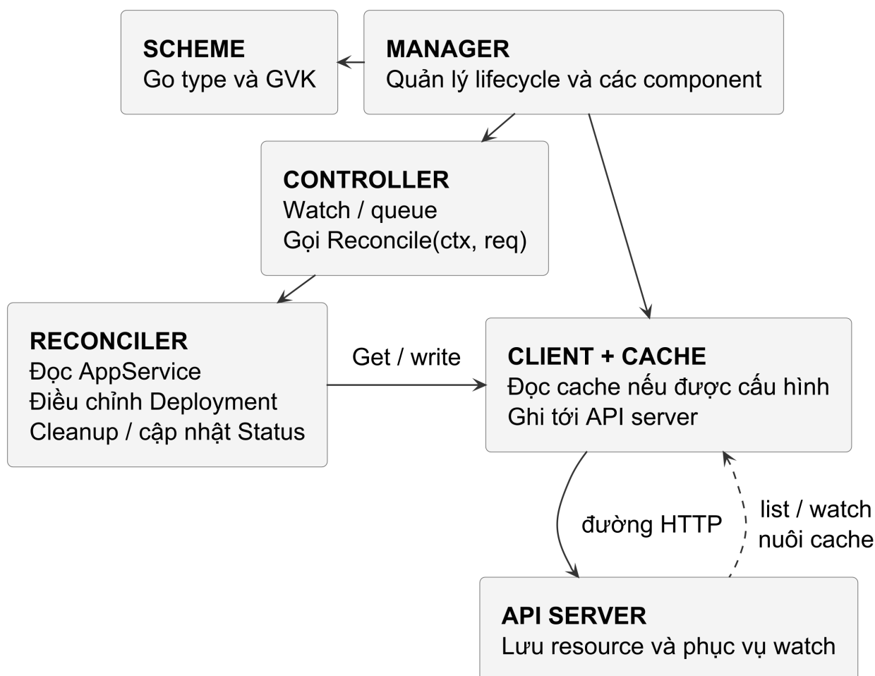
Hình 39 — Manager tổ chức các component; controller gọi Reconciler cho một khóa. Client dùng cache cho đường đọc được cấu hình và HTTP cho đường ghi; sơ đồ lược bỏ các đường đọc không qua cache.
