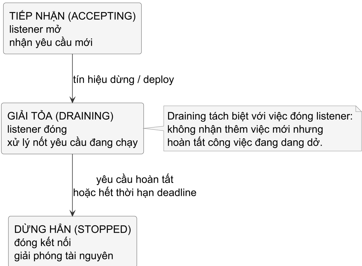
Hình 24 — Lifecycle khái niệm khi service graceful shutdown. Deadline của shutdown là policy vận hành: nó giới hạn thời gian chờ, không biến mọi request thành thành công.
