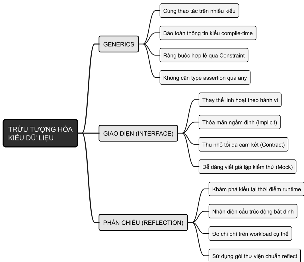
Hình 34 — Chọn abstraction theo câu hỏi cần trả lời. Sơ đồ là mental model, không mô tả representation runtime của interface hay cách compiler sinh code.
