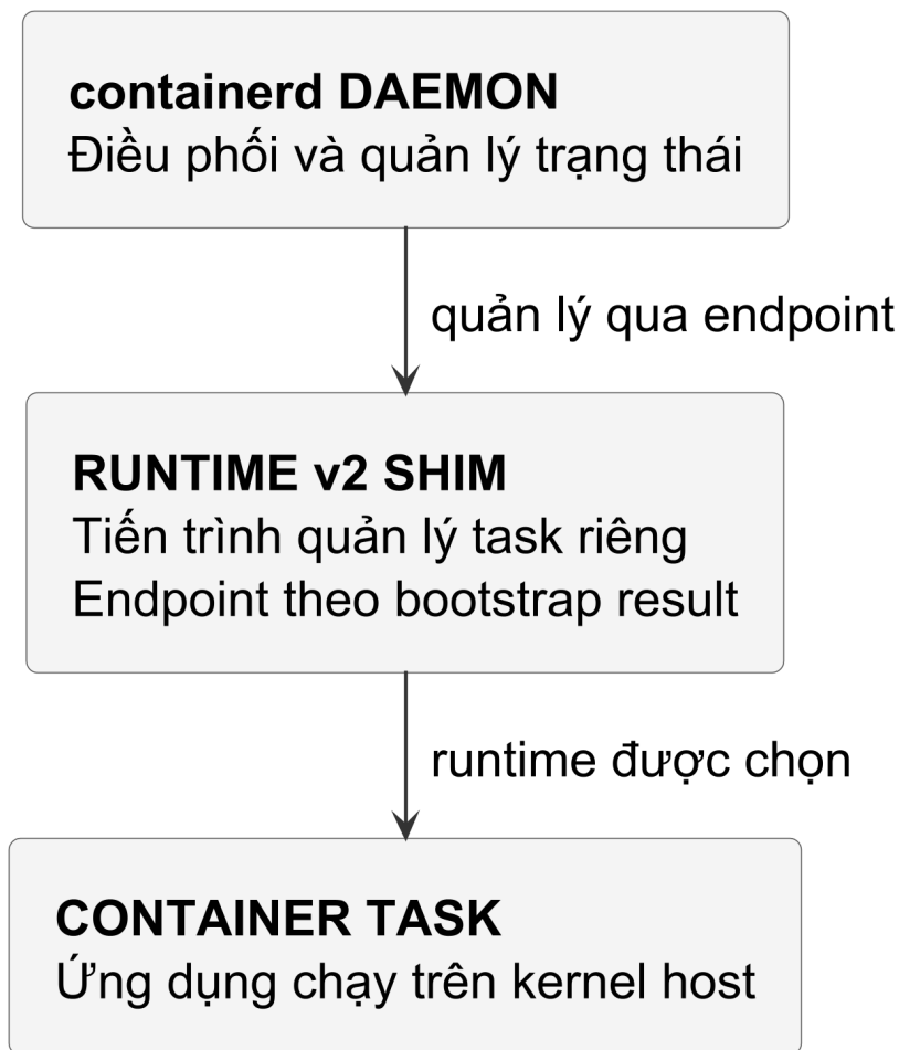
Hình 54 — Daemon giao tiếp với shim qua endpoint; shim quản lý task qua runtime được chọn. Ranh giới tiến trình này không bảo đảm mọi failure của daemon đều vô hại với workload.
