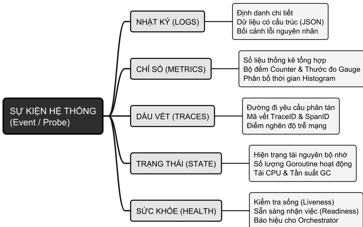
Hình 27 — Các signal trả lời các câu khác nhau. Diagram là mental model, không phải kiến trúc bắt buộc hay pipeline OpenTelemetry hoàn chỉnh.
