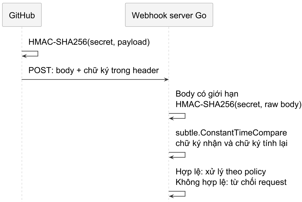
Hình 44 — Server tính chữ ký từ chính raw body đã nhận rồi so sánh với header. Không tuần tự hóa lại JSON trước khi kiểm tra chữ ký.
