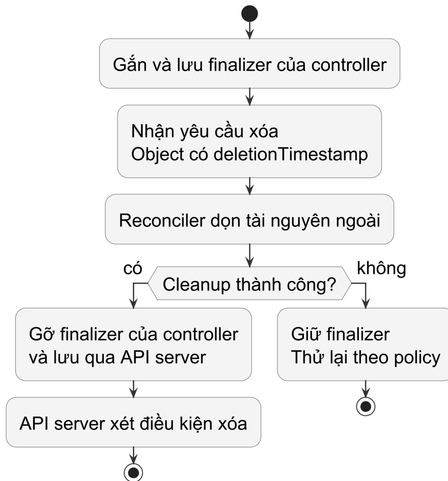
Hình 40 — Cleanup thất bại giữ finalizer để có thể thử lại. Cleanup thành công chỉ cho phép gỡ finalizer của controller này; API server còn phải xét các điều kiện xóa khác.
