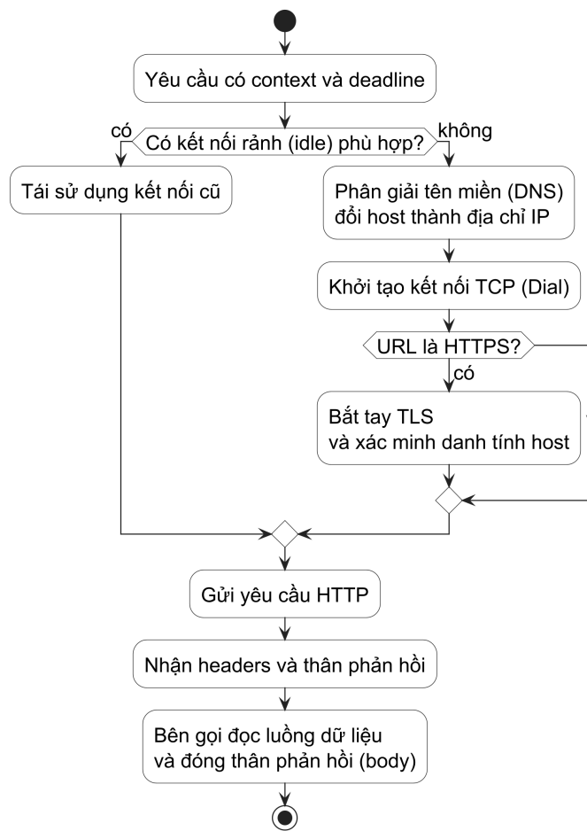
Hình 23 — Bản đồ khái niệm của một request client. Nhánh “connection idle” bỏ qua DNS, TCP và TLS mới; response body vẫn là tài nguyên caller phải hoàn tất vòng đời.
