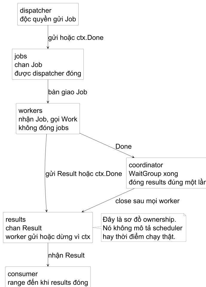
Hình 21 — Sơ đồ này là mental model về ownership, không phải timeline scheduler. Mỗi channel có một owner của tín hiệu kết thúc, và mọi đường worker phải có lối thoát khi consumer không còn nhận.
