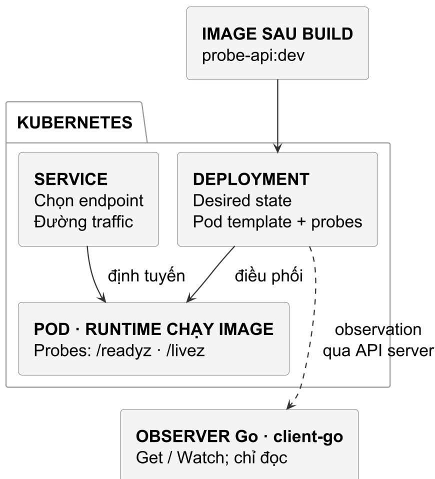
Hình 31 — Deployment khai báo Pod template cùng probes, Service chọn đường traffic, runtime trên node chạy image. Observer chỉ đọc qua API server; sơ đồ lược bỏ các component điều phối trung gian.
