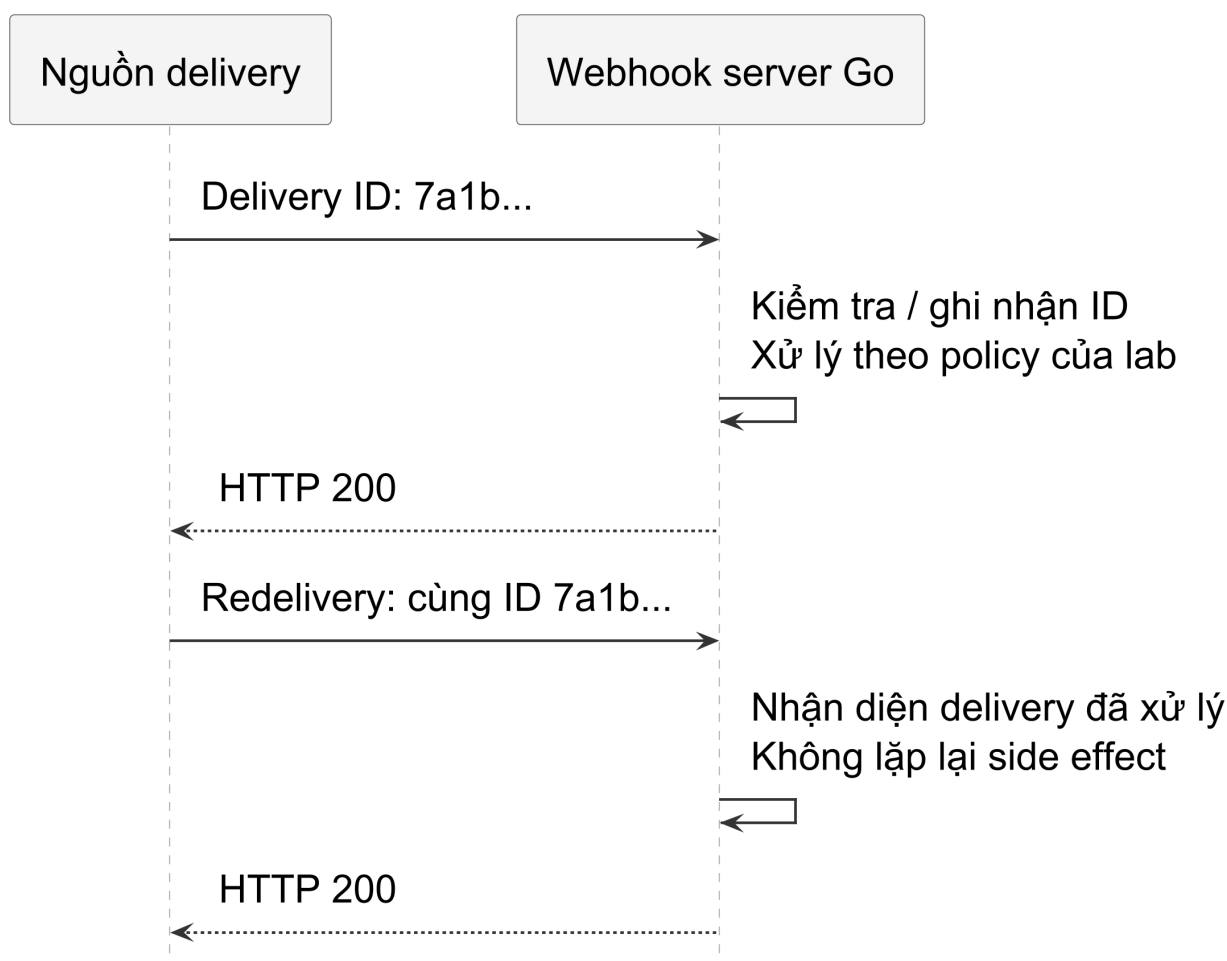
Hình 45 — Lab nhận diện cùng Delivery ID để tránh lặp side effect trong đường chạy được kiểm thử. Lưu bền, xử lý crash và delivery đồng thời cần policy cùng cơ chế riêng.
