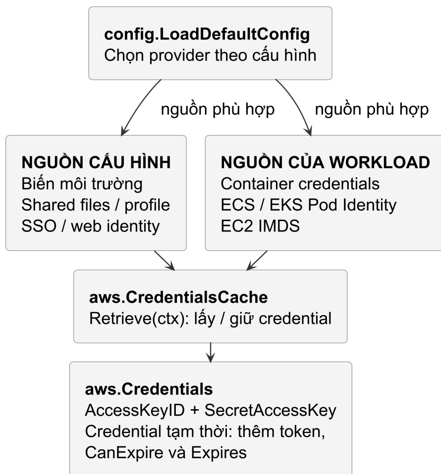
Hình 41 — Cấu hình quyết định provider được chọn; đây là bản đồ nguồn, không phải thứ tự ưu tiên bất biến. Credential có thể là static hoặc tạm thời. Cache lấy credential khi có lượt Retrieve cần dữ liệu hợp lệ.
