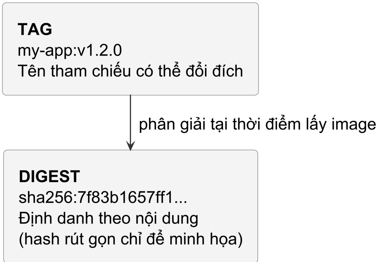
Hình 48 — Tag được phân giải thành digest tại một thời điểm. Dùng digest cố định nội dung được tham chiếu, không tự xác minh người tạo hay độ an toàn của nội dung ấy.
