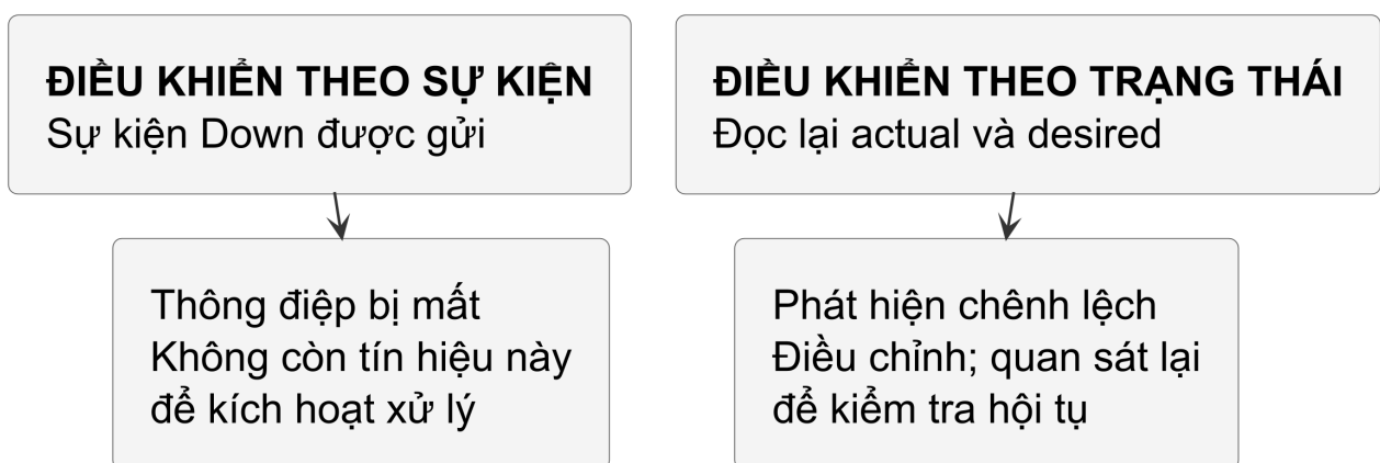
Hình 35 — Khi một thông điệp bị mất, controller dựa vào trạng thái có thể đọc lại observation và tiếp tục điều hòa. Khả năng hội tụ vẫn phụ thuộc việc quan sát và điều chỉnh thành công.
