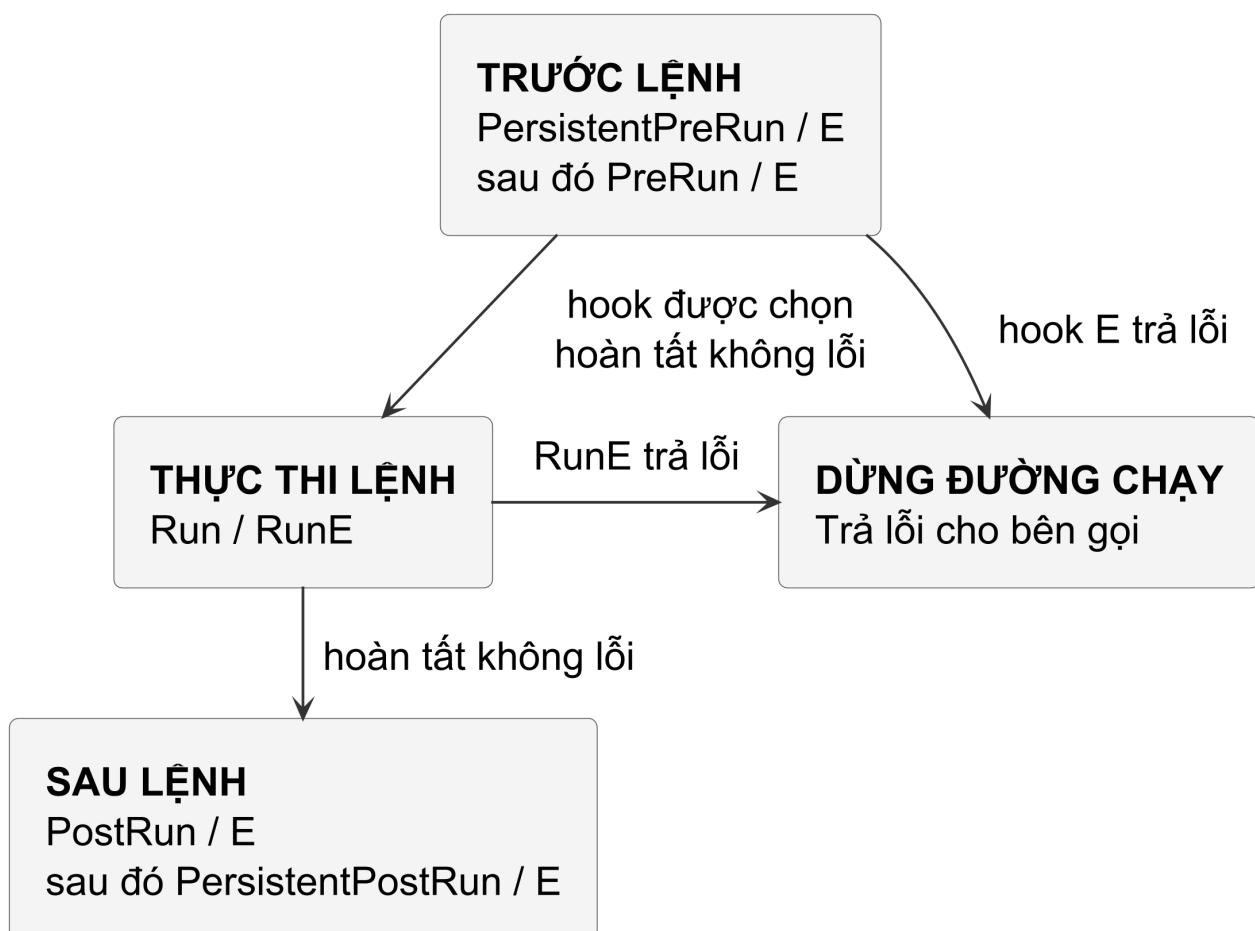
Hình 56 — Chỉ các hook được chọn mới chạy; hook có thể vắng. Lỗi từ hook E hoặc RunE ngắt đường chạy trước các hook phía sau.
