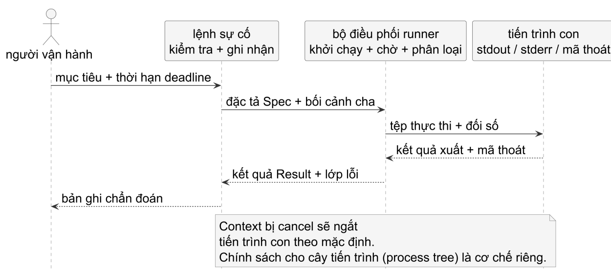
Hình 26 — Mô hình khái niệm. Result là bằng chứng cục bộ về một lần chạy; nó không tự chứng minh nguyên nhân gốc của incident.
