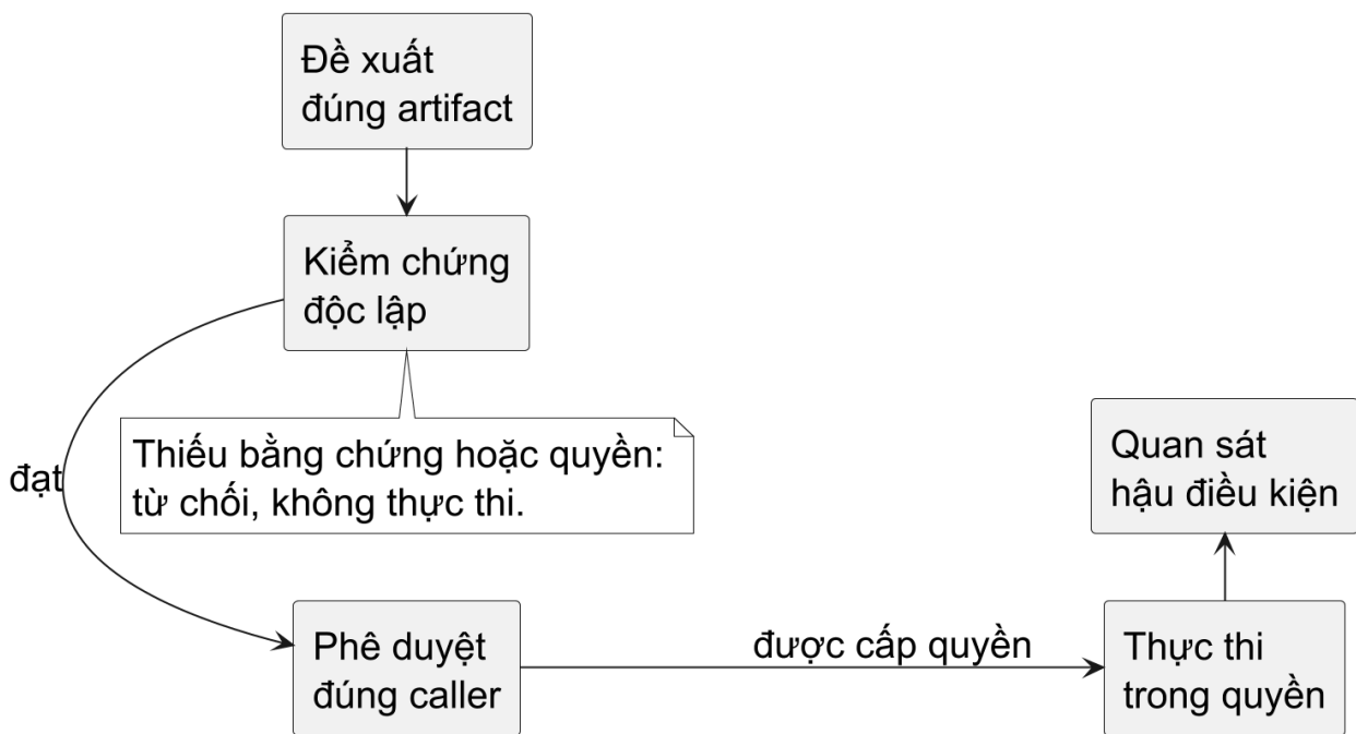
Hình 50 — Đề xuất không có quyền thực thi. Mỗi bước kiểm tra phải gắn với đúng artifact, target và caller; mỗi tên diễn tả policy của scenario, không phải một protocol đảm bảo an toàn sẵn có.
