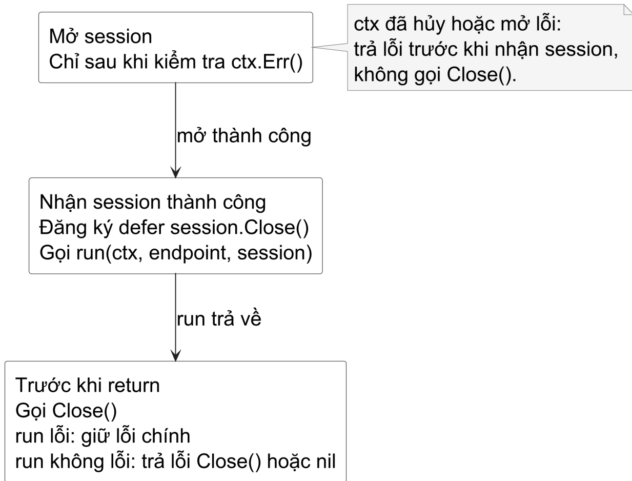
Hình 18 — defer không phải một câu thần chú dọn dẹp toàn chương trình. Nó ràng buộc cleanup với scope đã nhận ownership. Error từ Close chỉ thay result khi run chưa có failure để bảo toàn nguyên nhân chính.
