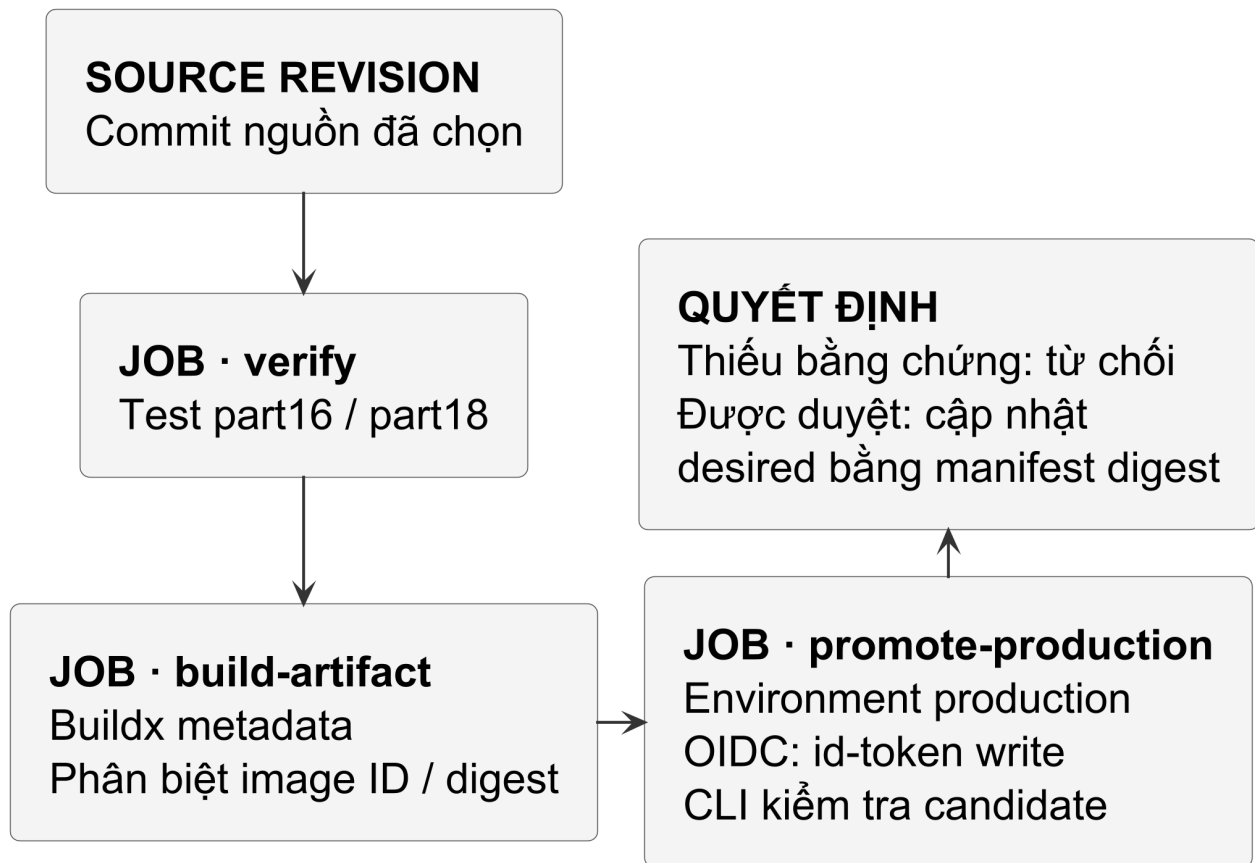
Hình 33 — Workflow truyền định danh và bằng chứng qua các job; quyền OIDC và environment không tự thay thế việc gate xác minh candidate. Chỉ quyết định được duyệt mới cập nhật desired state bằng digest.
