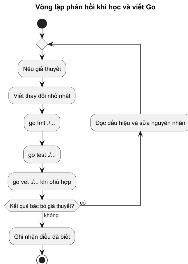
Hình 3 — Vòng lặp phản hồi giả thuyết - đo đạc - sửa mã nguồn. Trình biên dịch không phải là chướng ngại vật; trình biên dịch là công cụ kiểm định tĩnh sớm nhất cho các dự đoán của bạn.
