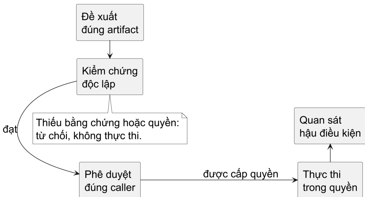
Hình 31 — Đề xuất không có quyền thực thi. Mỗi bước kiểm tra phải gắn với đúng artifact, target và caller; mỗi tên diễn tả policy của scenario, không phải một protocol đảm bảo an toàn sẵn có.
