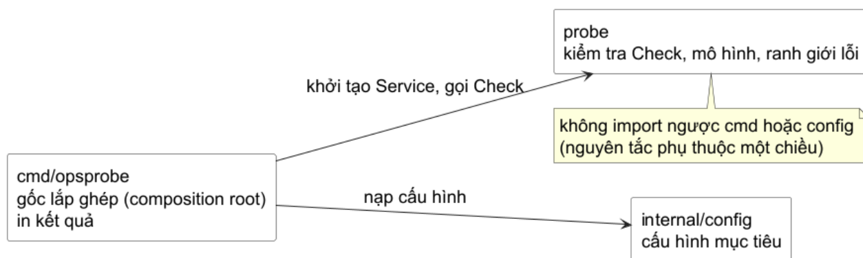
Hình 19 — Dependency direction là công cụ review. cmd/opsprobe là composition root ; nó biết các package cụ thể. probe không biết CLI hay config source nên có thể được đọc, test và thay thế runner mà không kéo presentation theo.
