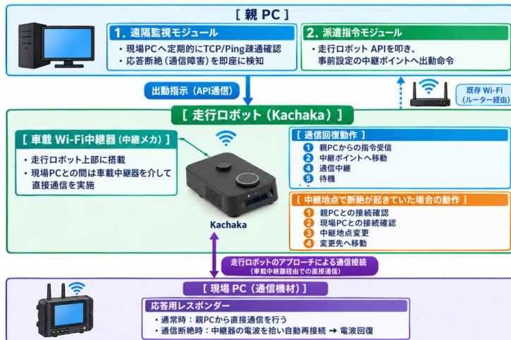
親PC・走行ロボット・現場PCの構成
