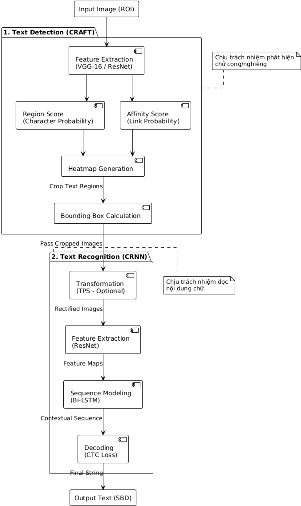
Hình 2.1: Sơ đồ kiến trúc đường ống xử lý của EasyOCR: Từ phát hiện (Detection) đến nhận dạng (Recognition)
