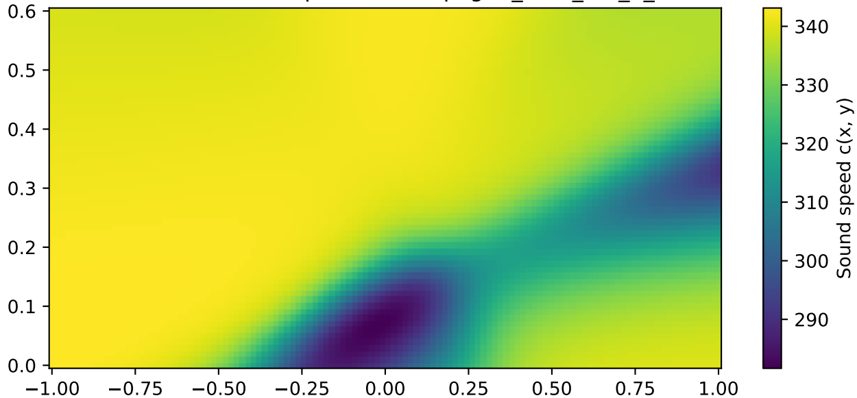
Phase 2 Adam snapshot 30% - pkg01_f600_m0_1_2
