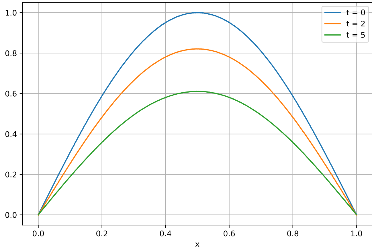
PINN
