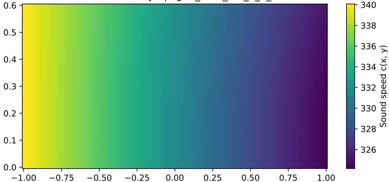
Inverted celerity - pkg01_f600_m0_1_2_3
