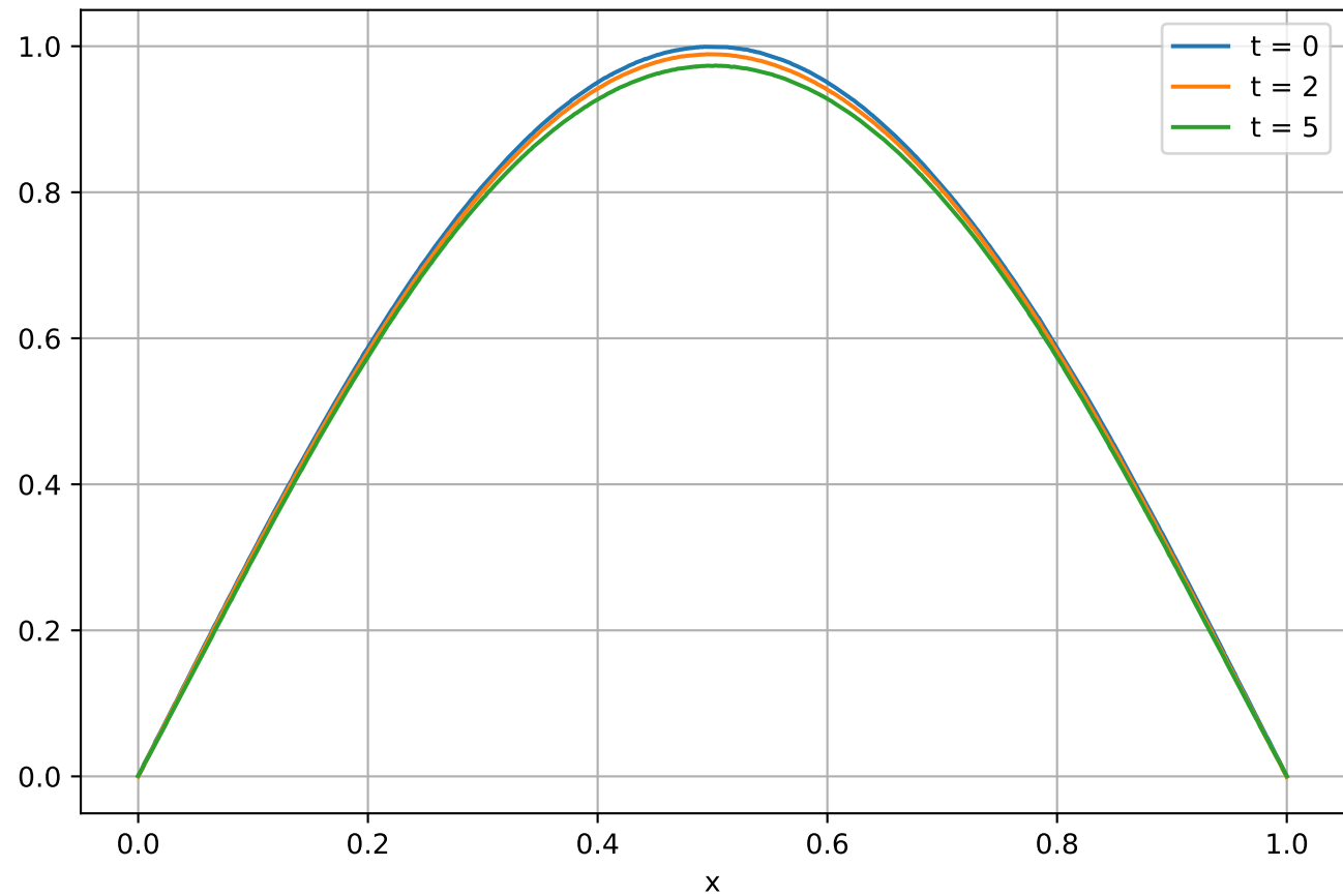
PINN
