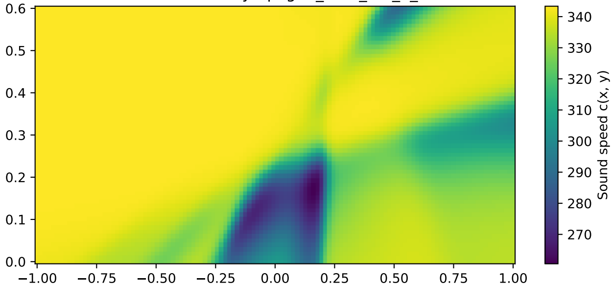
Inverted celerity - pkg01_f600_m0_1_2
