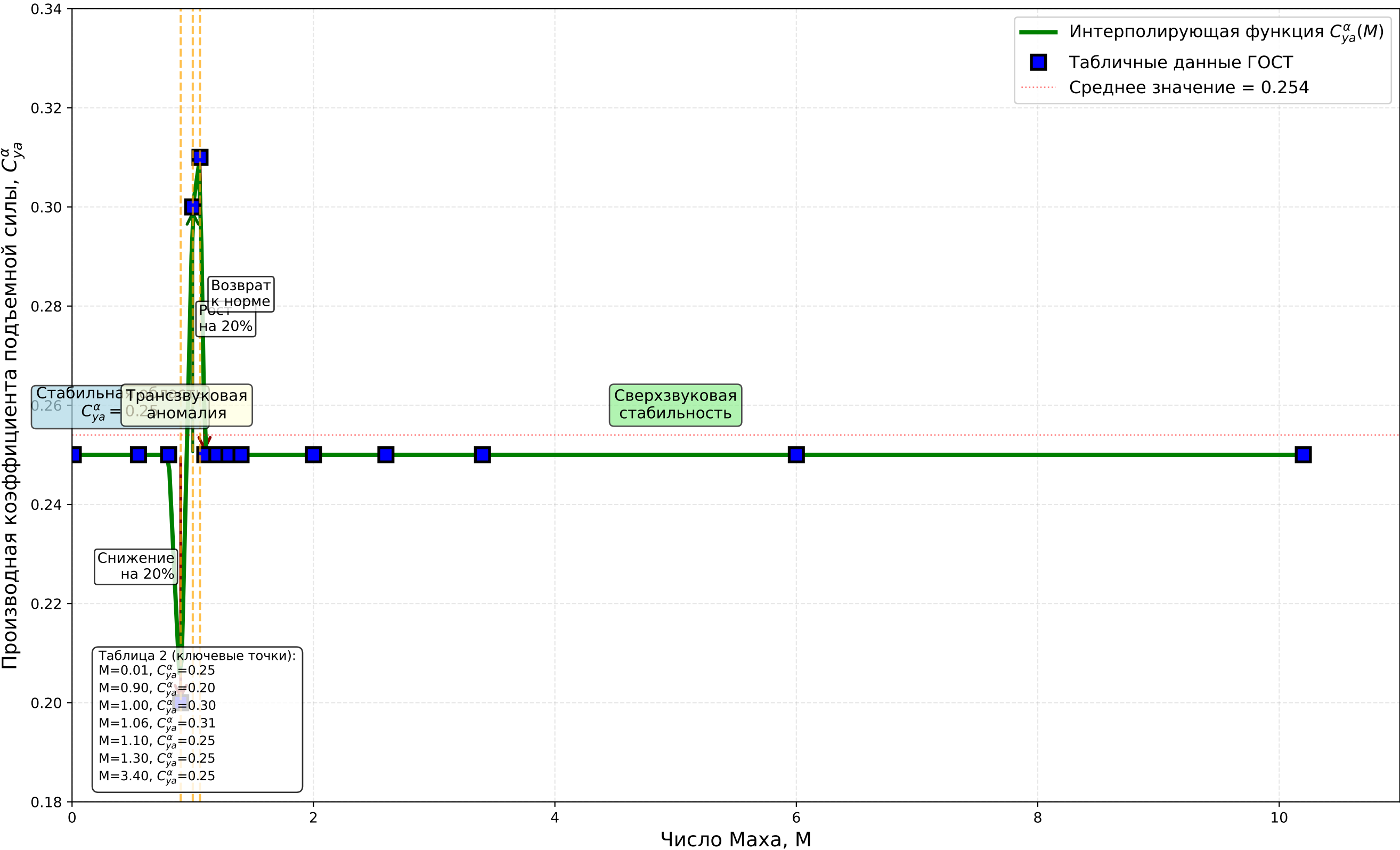
Зависимость производной коэффициента подъемной силы от числа Маха C_{ya}^{\alpha}(M)
