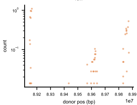
raw
