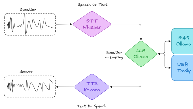
Figura 4.1: Estructura del sistema del asistente de voz usando modelos locales para cada fase.
