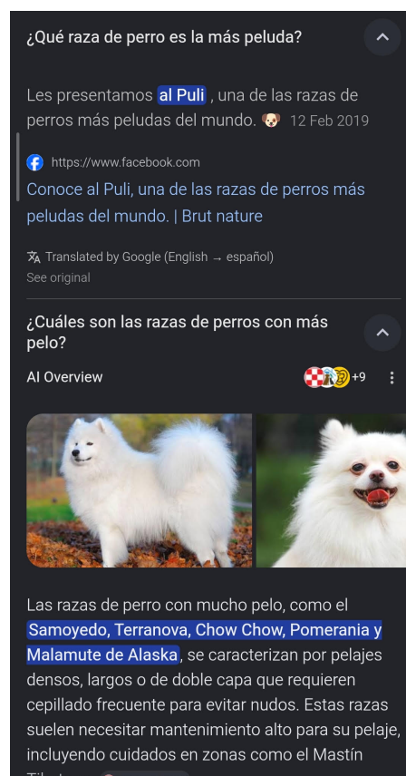
Figura 5.2: Ejemplo de inconsistencia en el sistema RAG, donde el evaluador prefiere buscar en la web ignorando los datos locales explícitamente disponibles.
