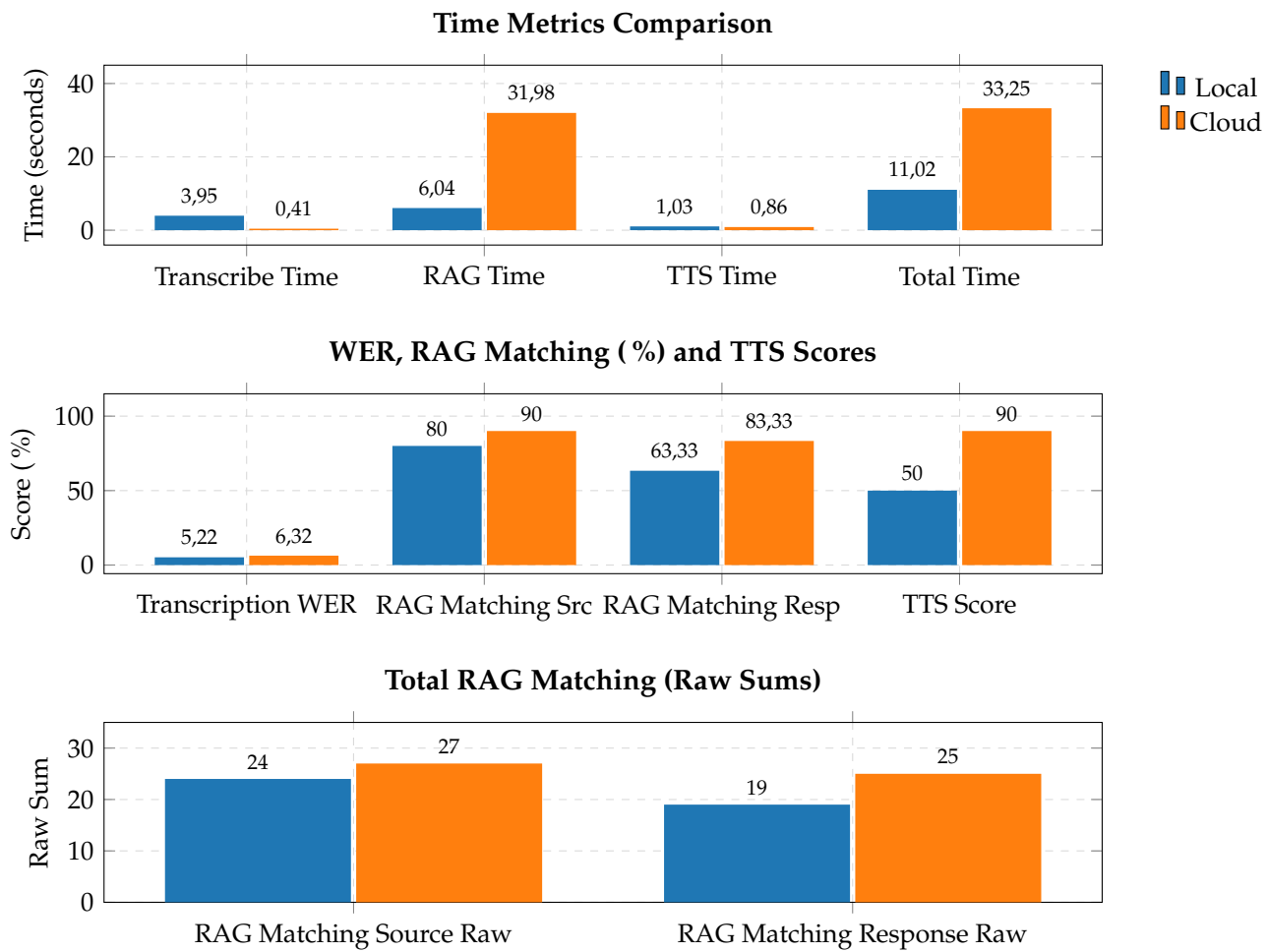
Figura 5.1: Visualización gráfica del contraste de resultados (Tiempos, % de acierto y Conteo Crudo).
