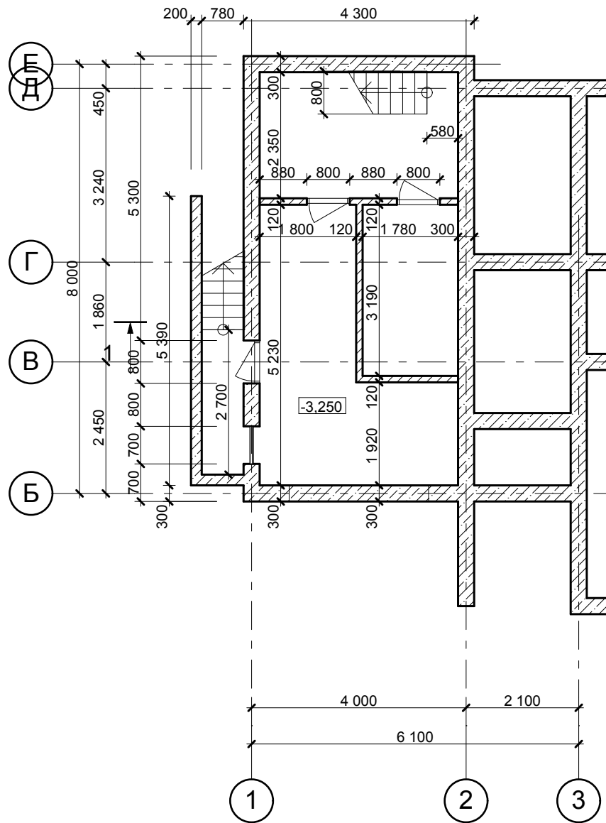
Кладочный план подвала
