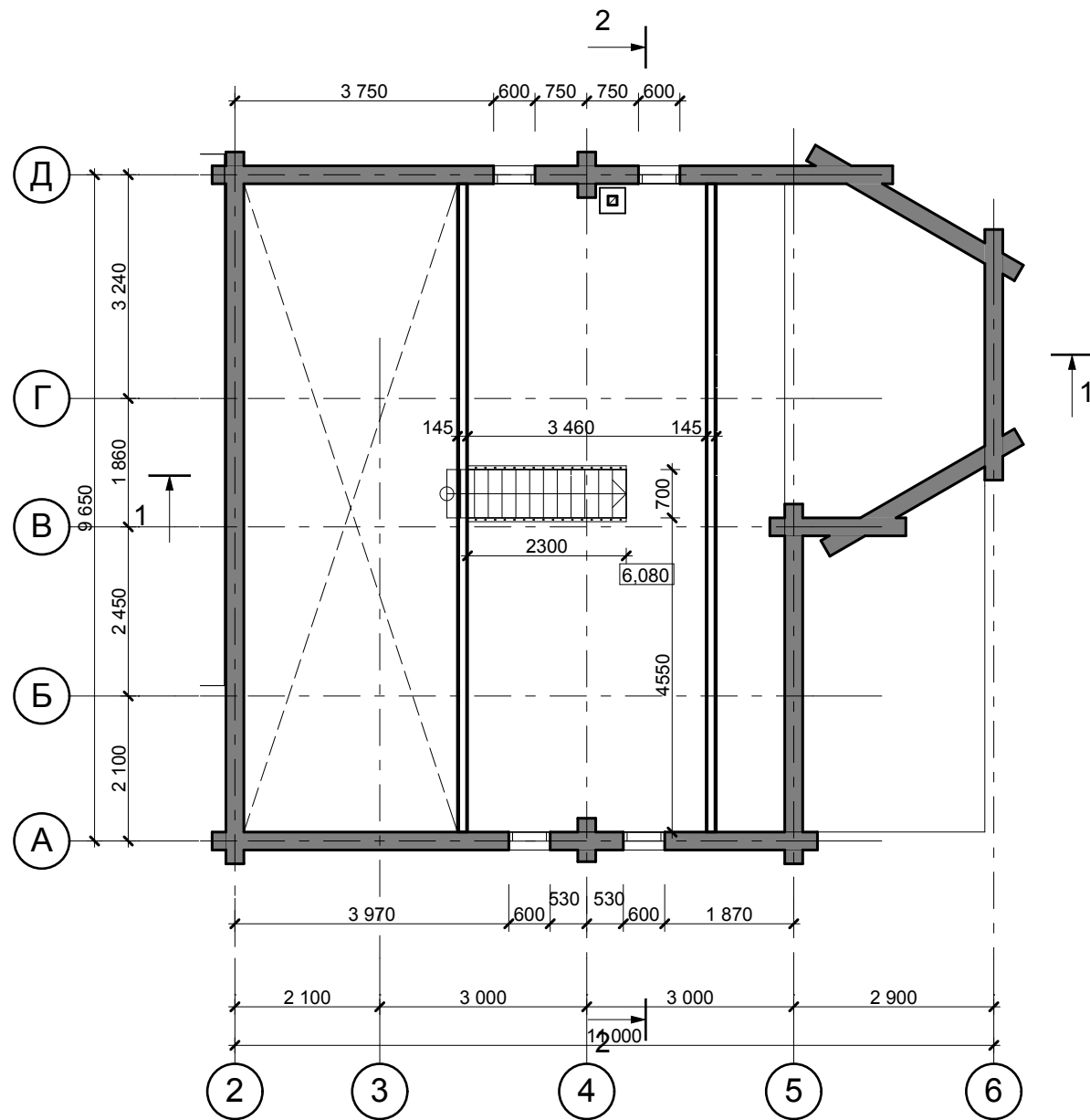
Кладочный план на отметке +6,080
