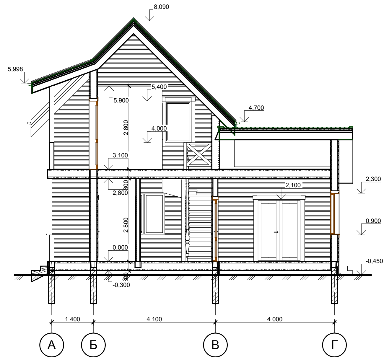
Разрез 2-2 (М 1:75)
