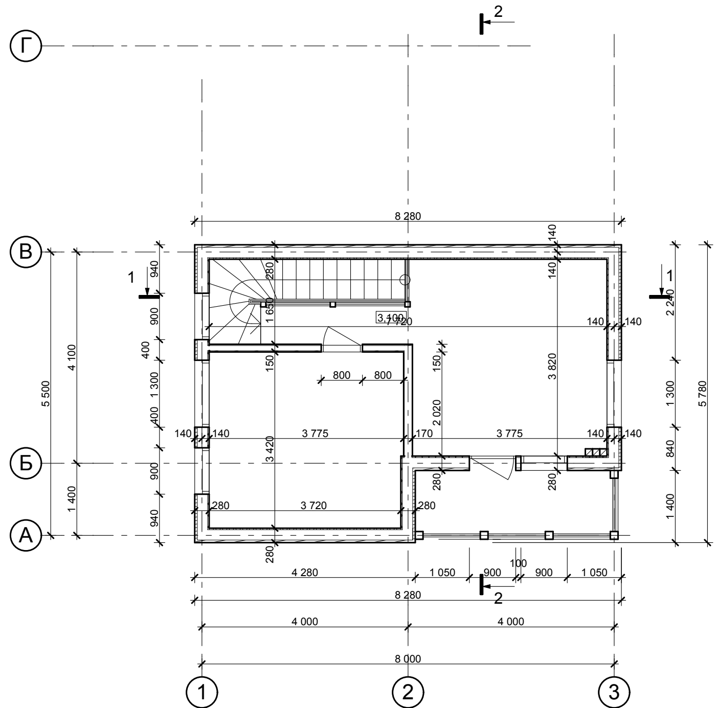
Кладочный план 2-го этажа (М 1:75)
