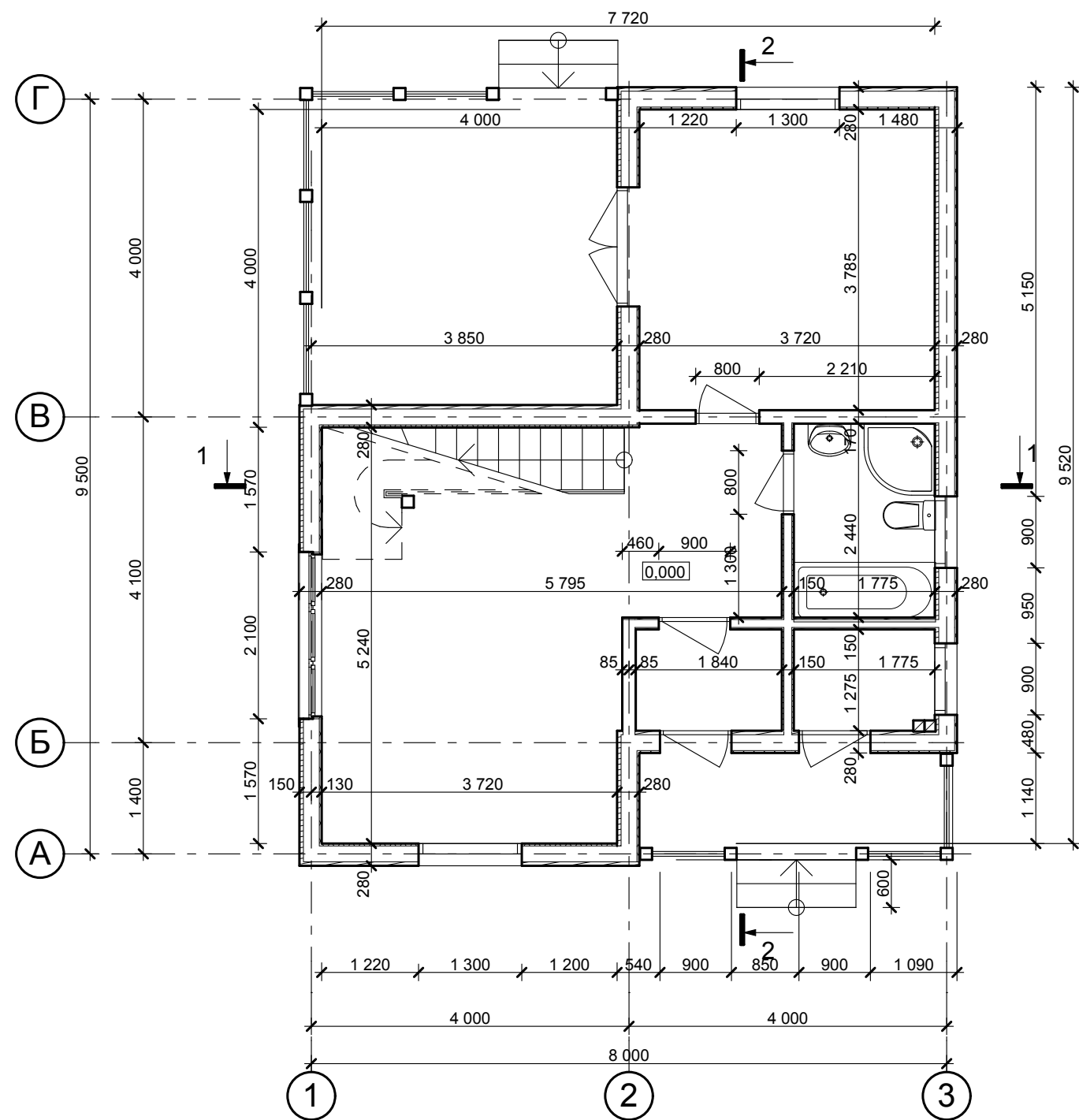
Кладочный план 1-го этажа (М 1:75)
