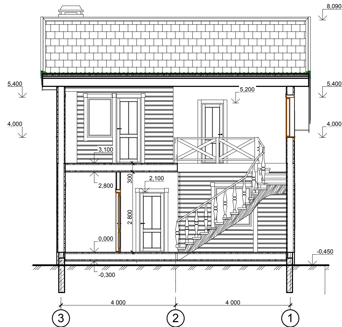
Разрез 1-1 (М 1:75)
