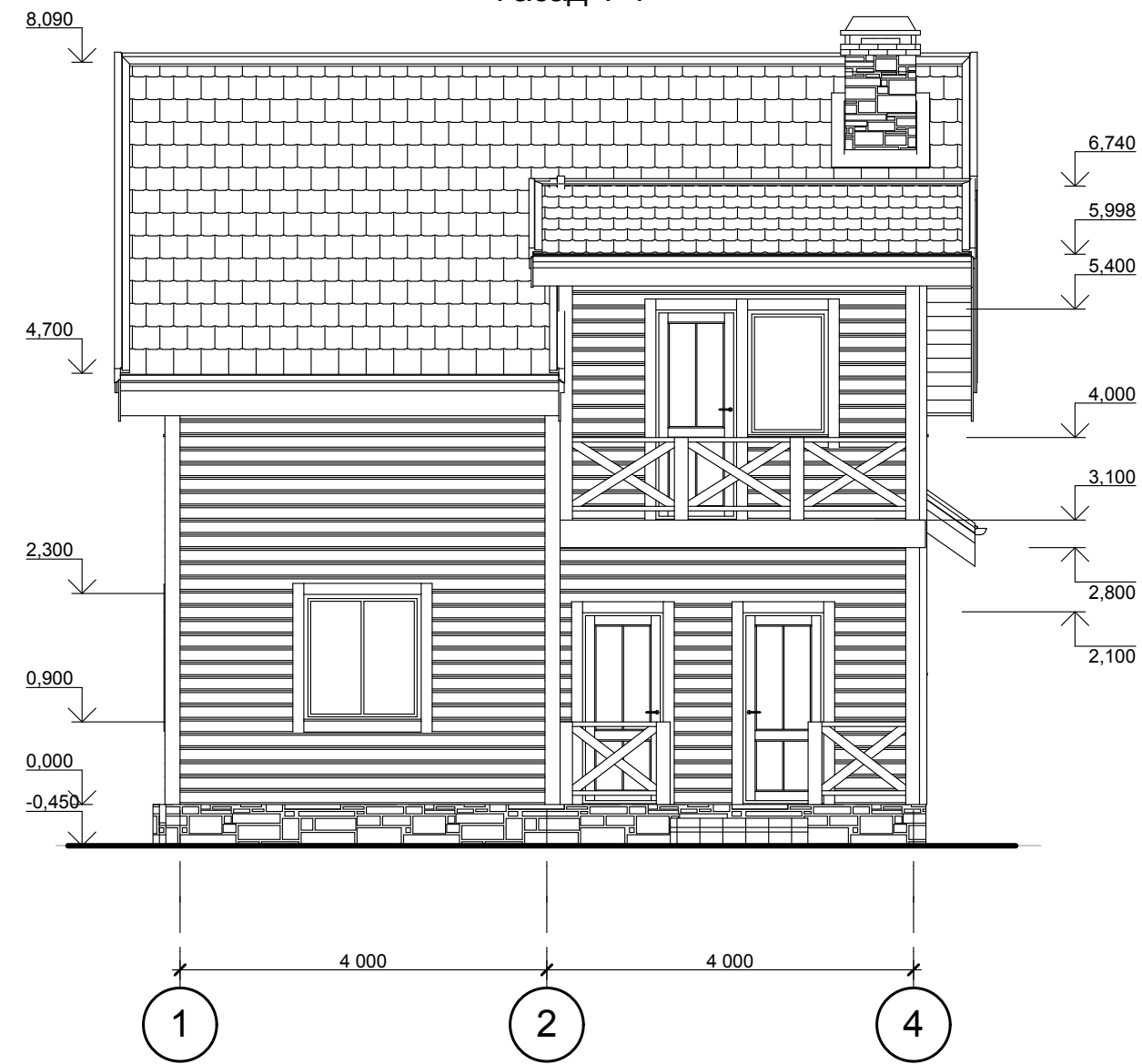
Фасад 1-4
