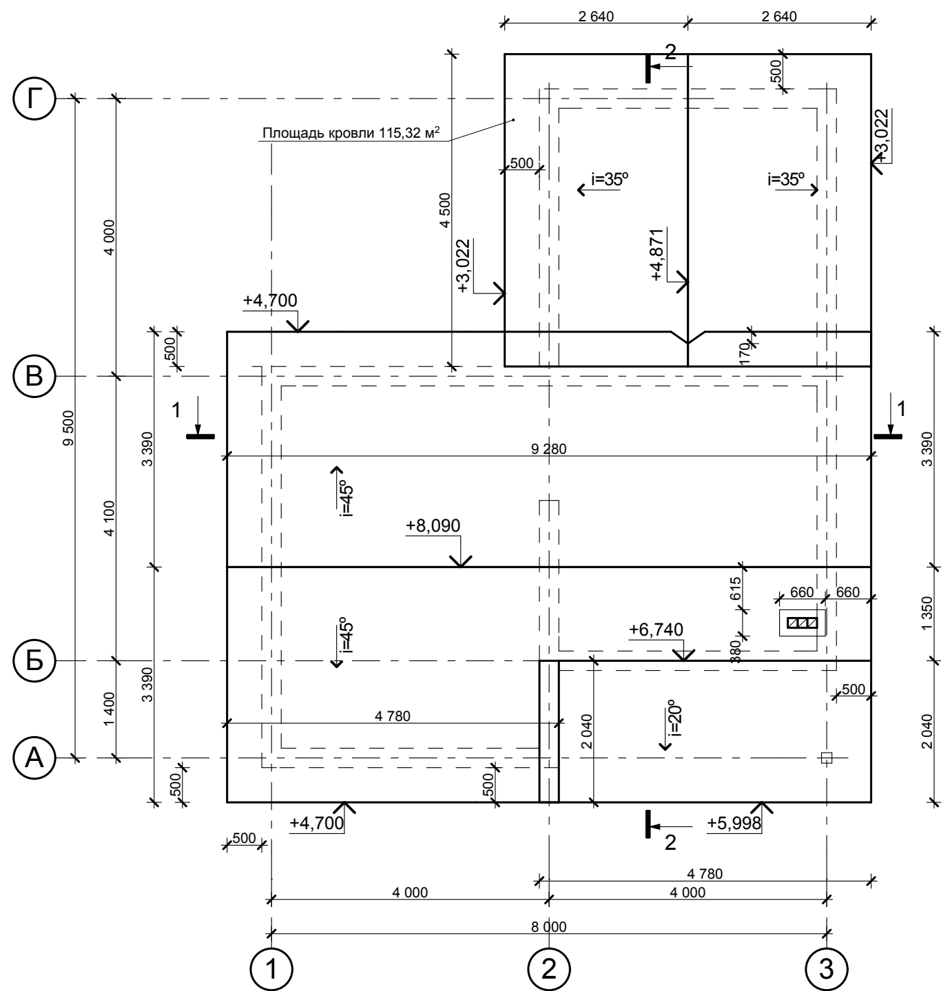
План кровли (М 1:75)
