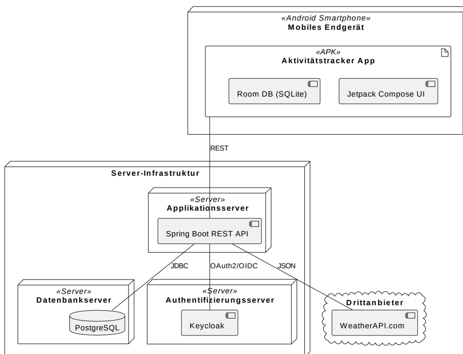
Abbildung 2.3: Deployment-Diagramm der Verteilungssicht
