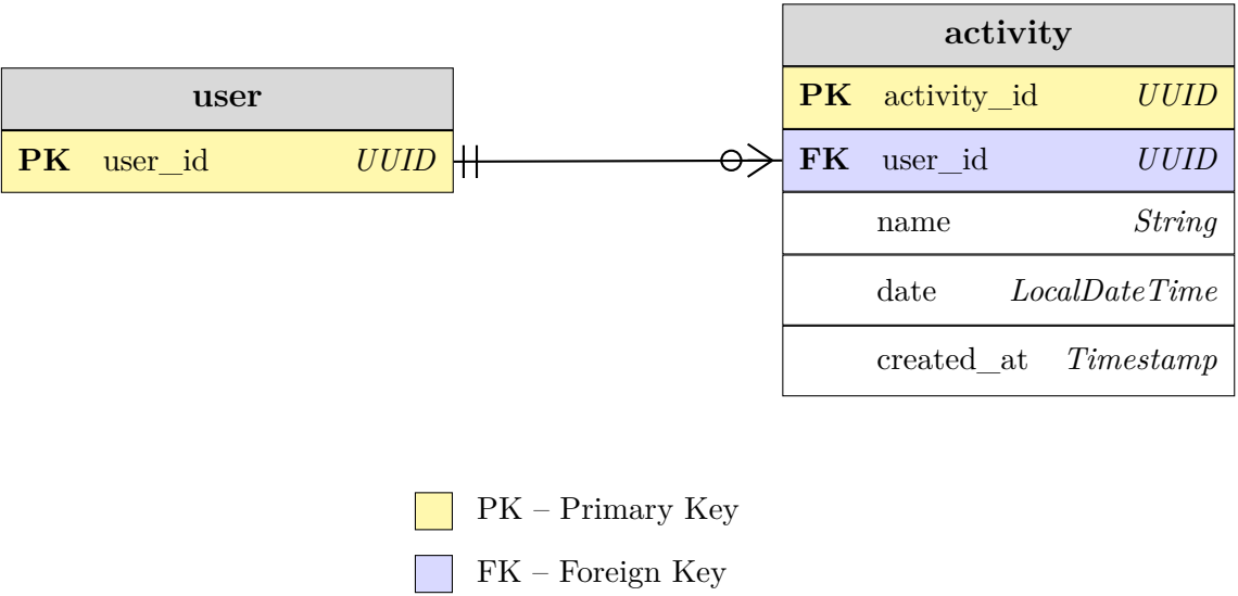
Abbildung 2.5: Physisches Datenmodell
