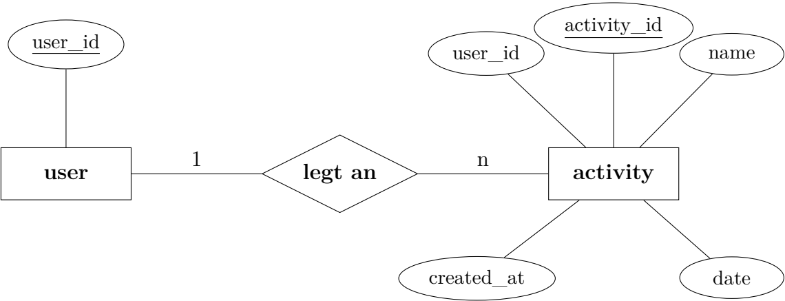
Abbildung 2.4: Konzeptionelles ER-Modell
