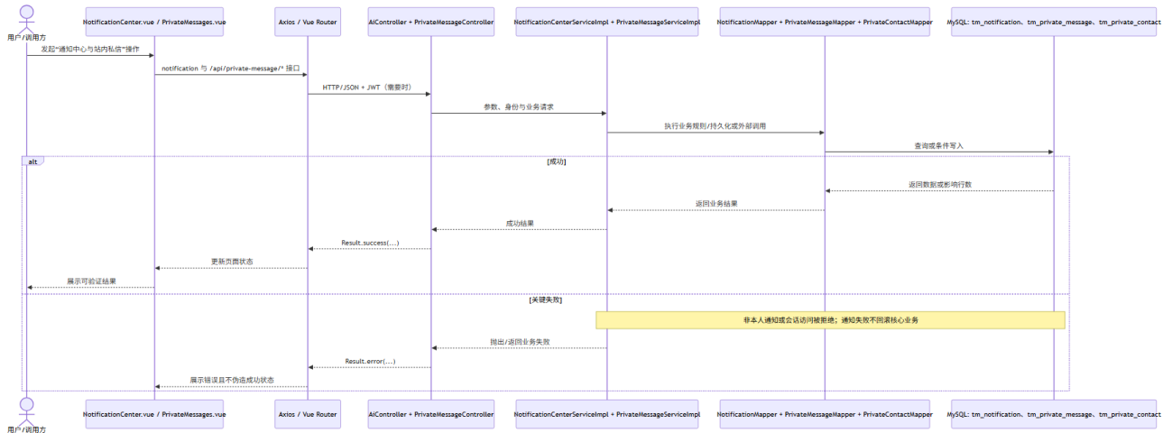
COMP-UC13 通知中心与站内私信——组件级顺序图
