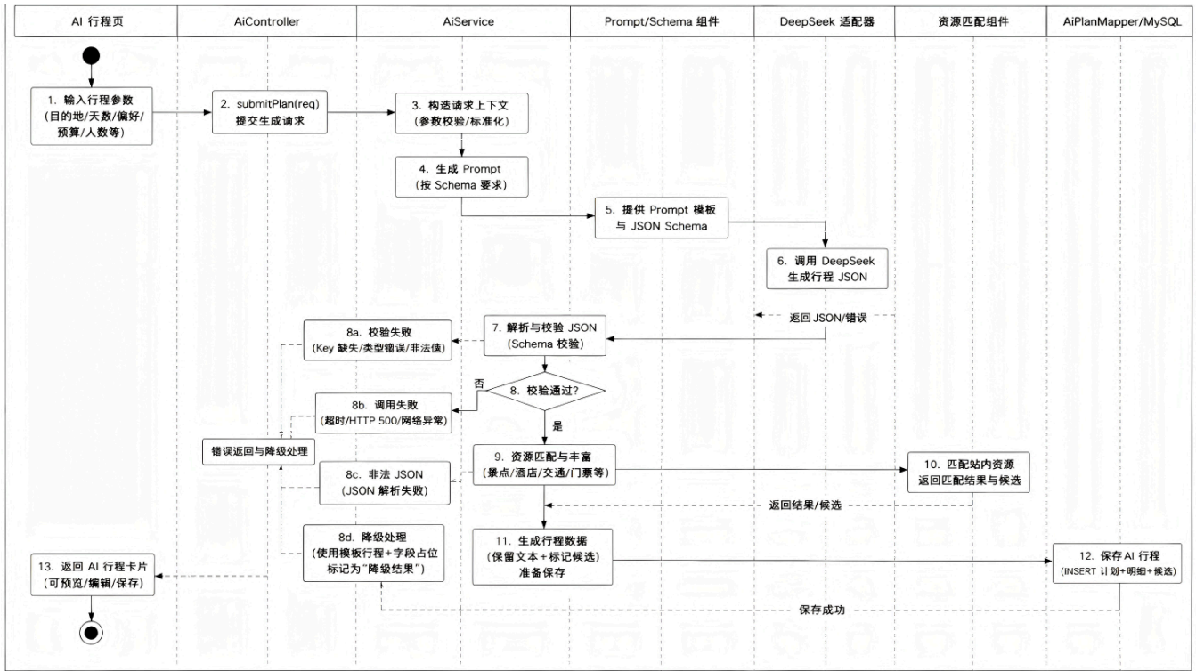
图 HLD-FIG-12 COMP-UC11 生成并保存 AI 行程组件级顺序图
