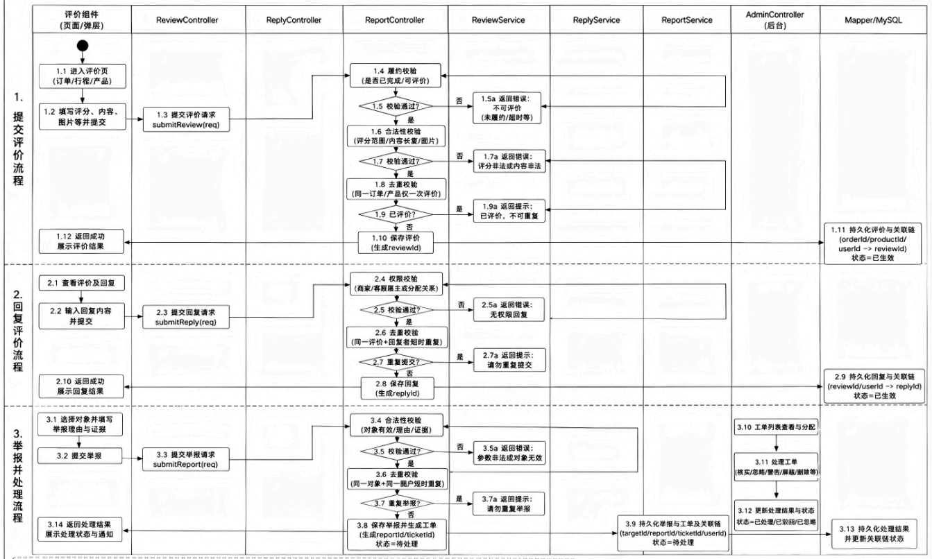
图 HLD-FIG-10 COMP-UC09 提交评价、回复评价与举报处理组件级活动图
