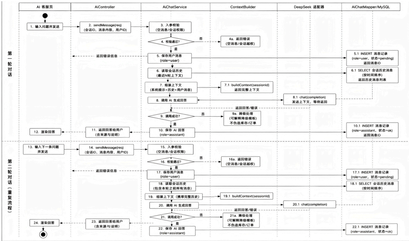
图 HLD-FIG-13 COMP-UC12 AI 客服多轮对话组件级顺序图
