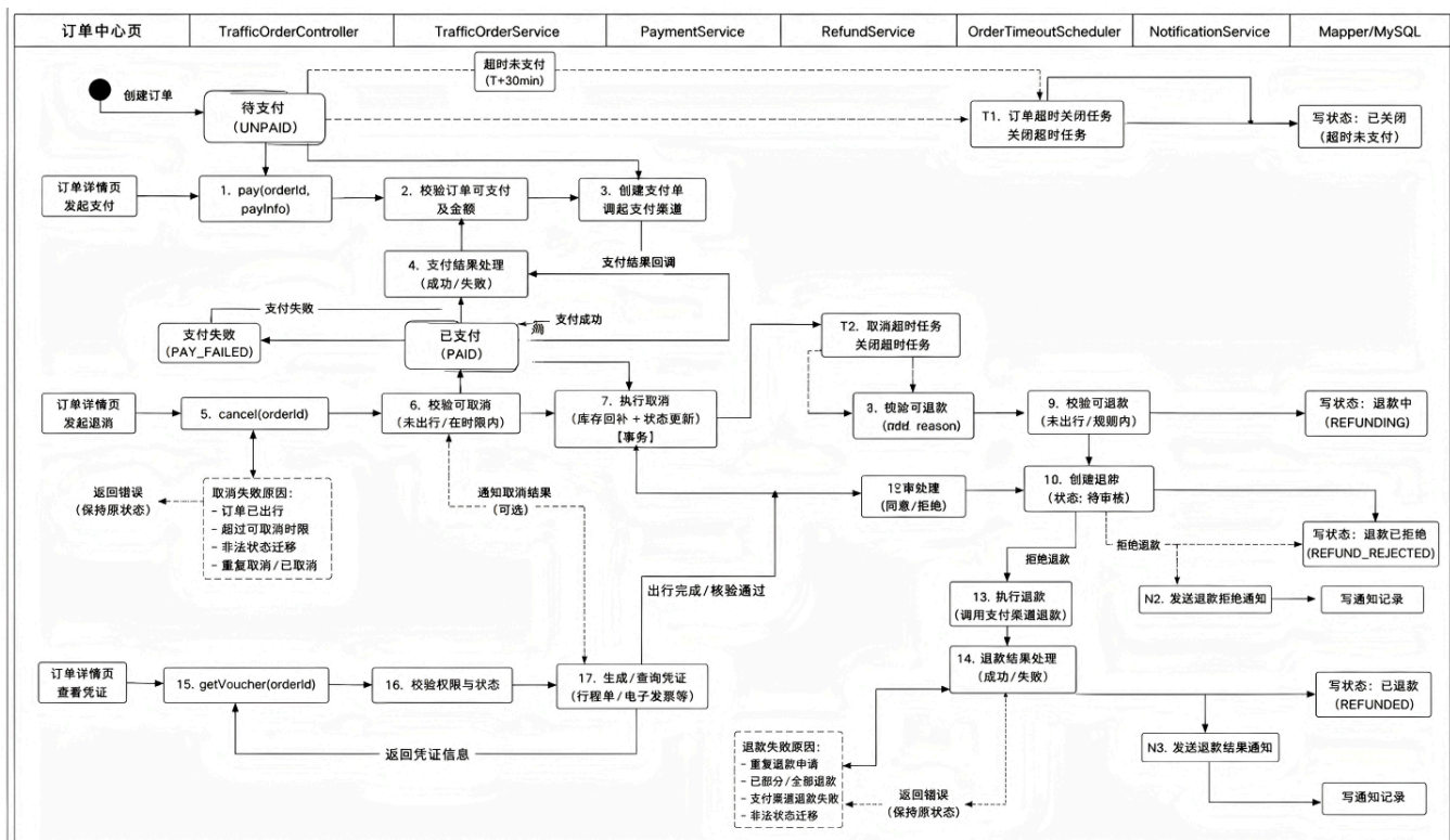
HLD-FIG-05 COMP-UC04 交通订单支付、取消、退款与凭证查看组件级状态图
