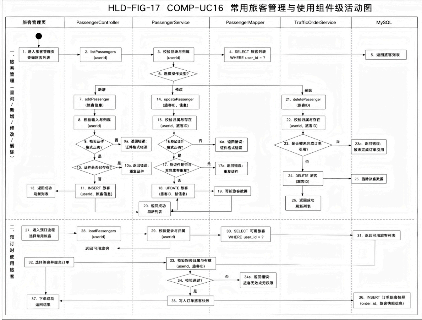
图 HLD-FIG-17 COMP-UC16 常用旅客管理与使用组件级活动图
