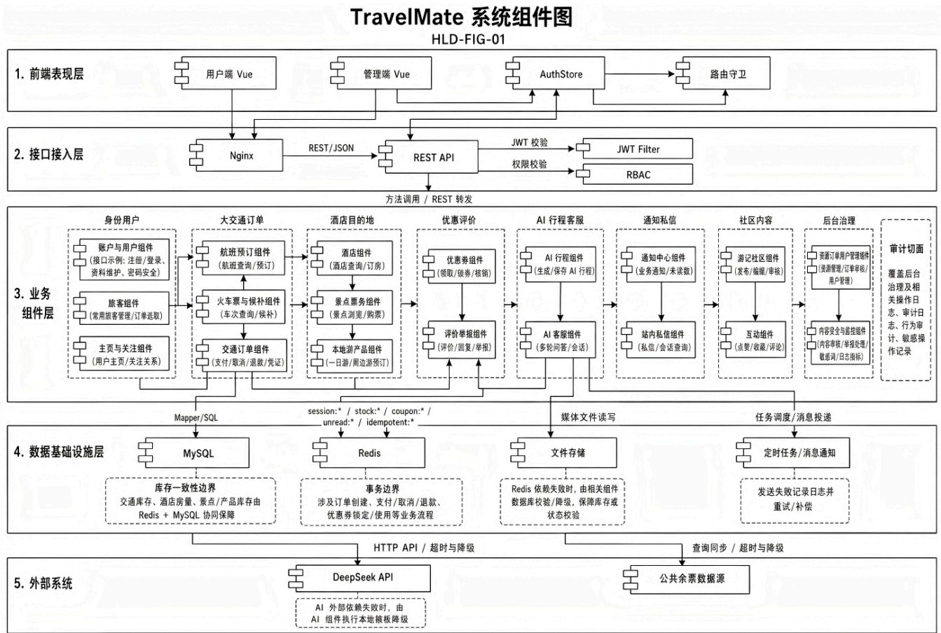
图 HLD-FIG-01 TravelMate 系统组件图
