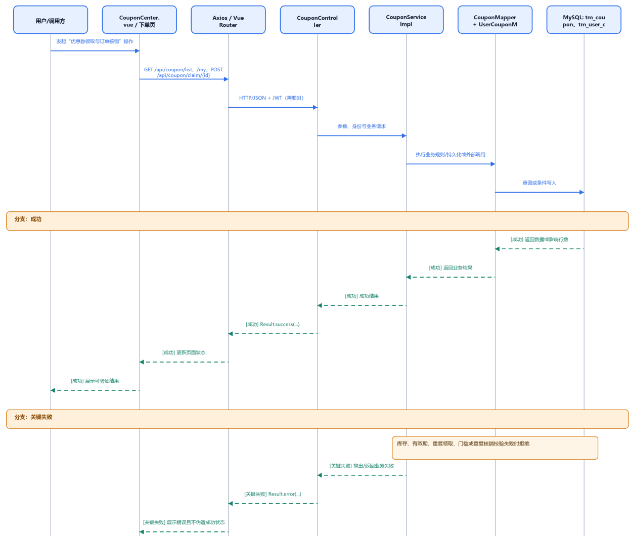
COMP-UC10 优惠券领取与订单核销——组件级顺序图 当前实现模型 | 成功、失败、权限、事务与幂等边界
