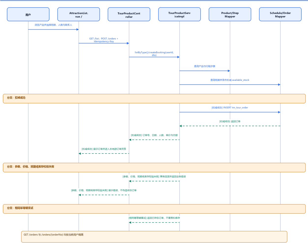
图 HLD-FIG-09 COMP-UC08 选择并预订一日游或周边游产品组件级活动图
