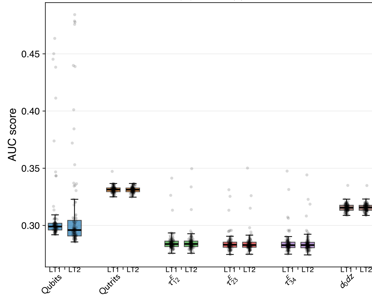
(b) W \rightarrow q\bar{q}
