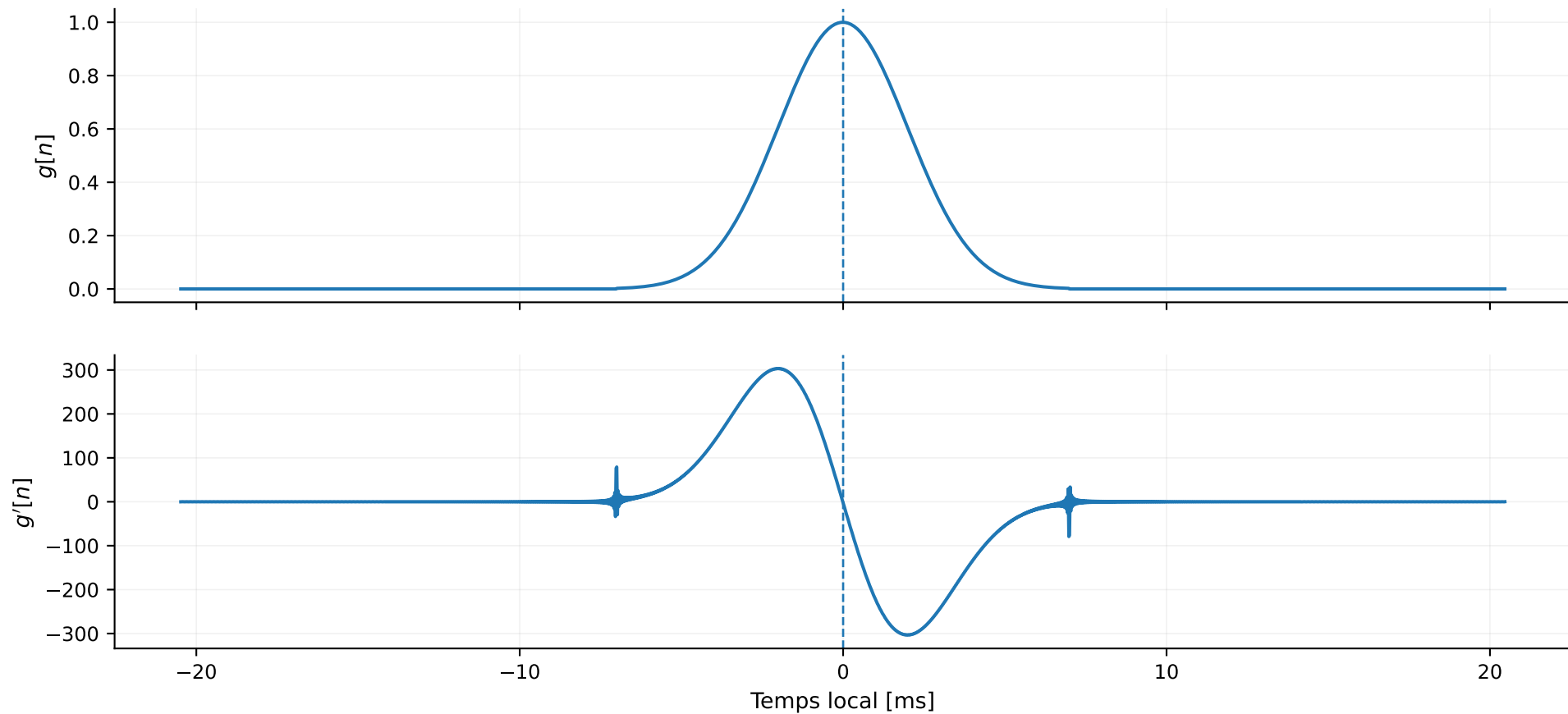
Figure 2 — Fenêtre gaussienne et fenêtré dérivée
