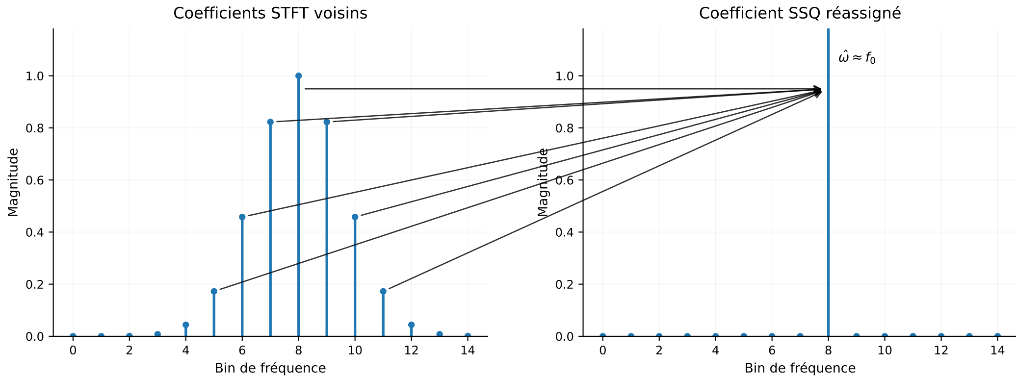
Figure 6 — Principe de réassignation dans le synchrosqueezing
