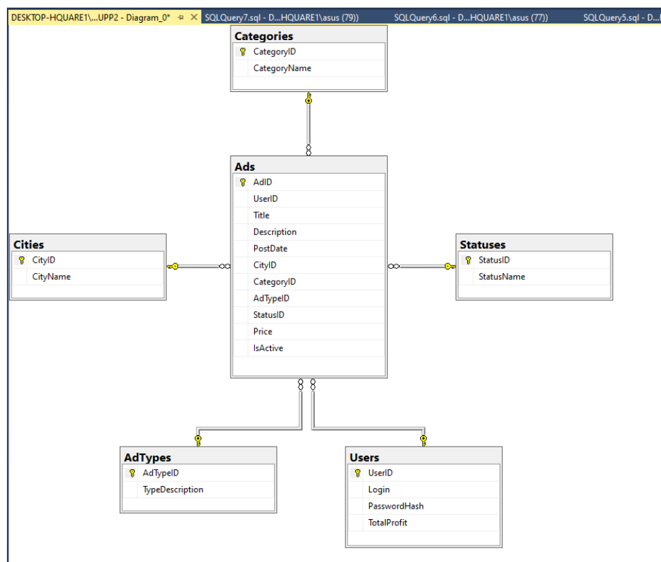
Рисунок 13 – ER-диаграмма
