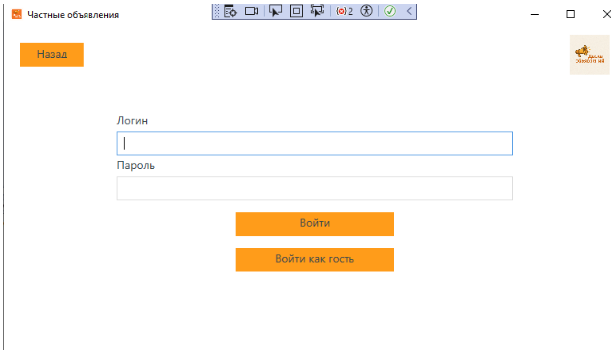
Рисунок 18 – Страница авторизации
