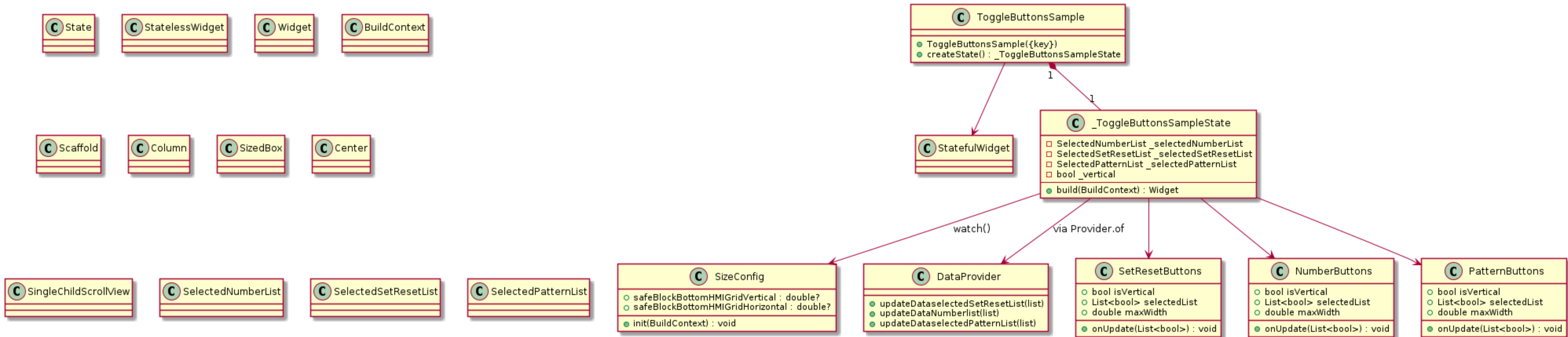
ToggleButtonsSample Class Diagram
