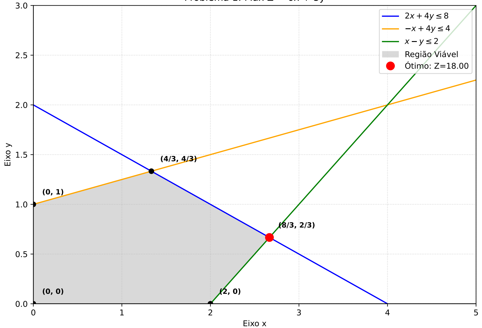
Problema 1: Max Z = 6x + 3y
