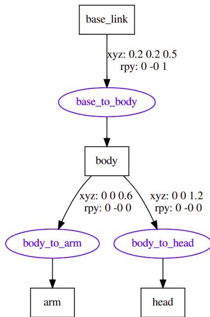
Рис. 1. URDF Tree (автоматический можно получить автоматически. Для создания читать здесь ).
