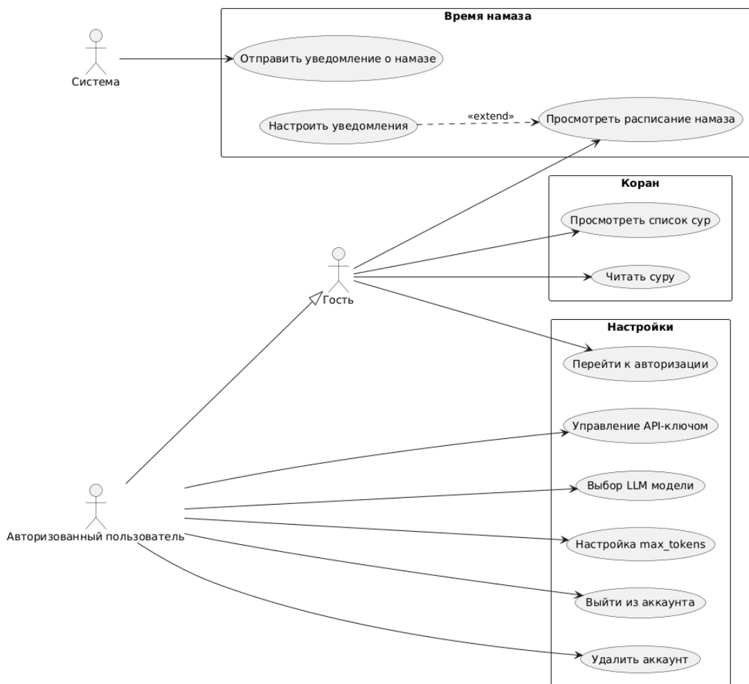
Рис.1.7. Use Case-диаграмма модулей "Коран "Время намаза"и "Настройки"
