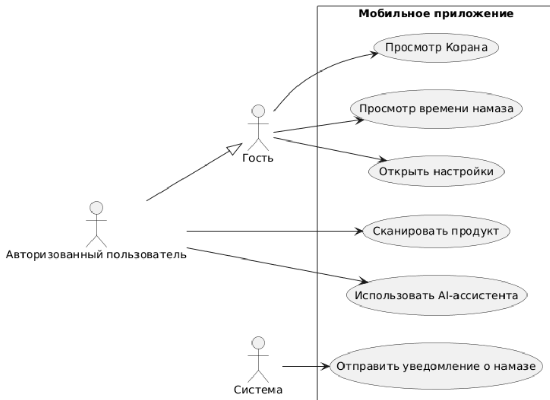
Рис.1.3. Общая диаграмма вариантов использования системы
