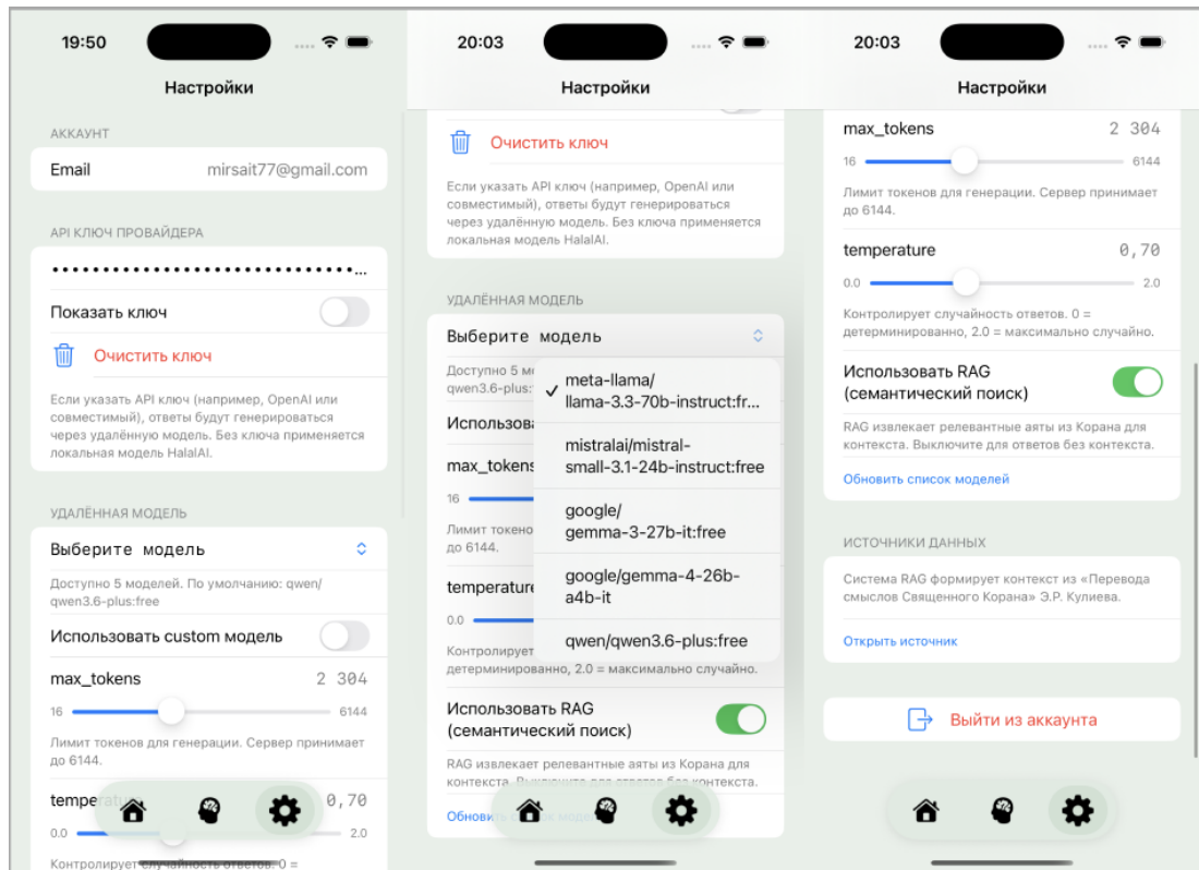
Рис.1.22. Макет экрана настроек
