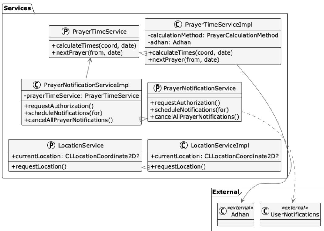
Рис.2.15. UML-диаграмма классов модуля времени молитвы. Services
