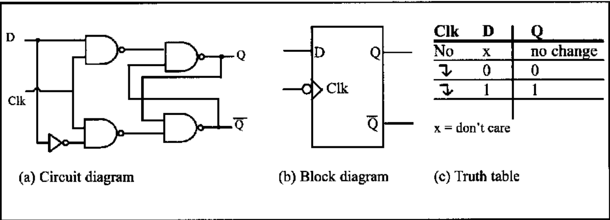
Figure 0-8. D Flip-Flops
