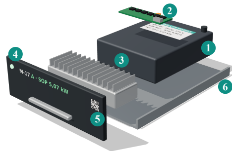
Gambar 4 - Isi satu laci: (1) modul EV bekas, (2) BMS, (3) DC/DC dua arah terisolasi 6 kW, (4) panel depan dengan LED kelas modul, (5) kode QR SOP passport , (6) nampan geser
