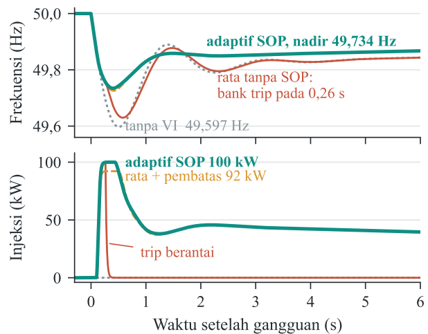
Gambar 5 - Frekuensi sistem dan daya injeksi VI untuk gangguan 250 kW pada model representatif ( H = 1,5 s)
