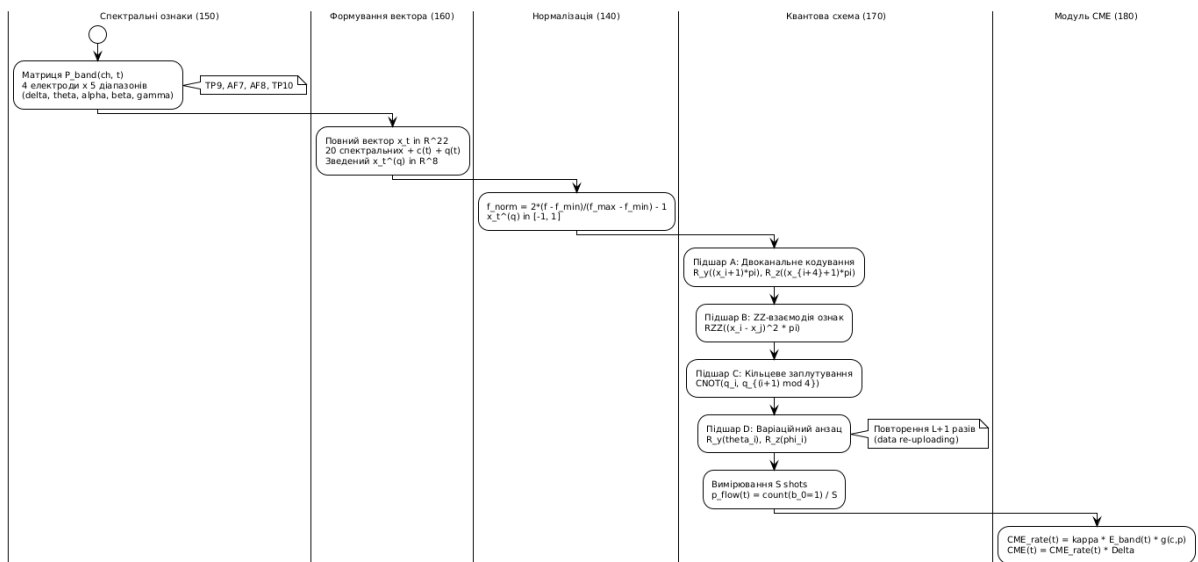
Фіг. 4 – Структура спектральних ознак
