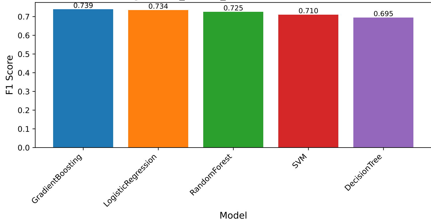
german_credit_data: Model vs F1
