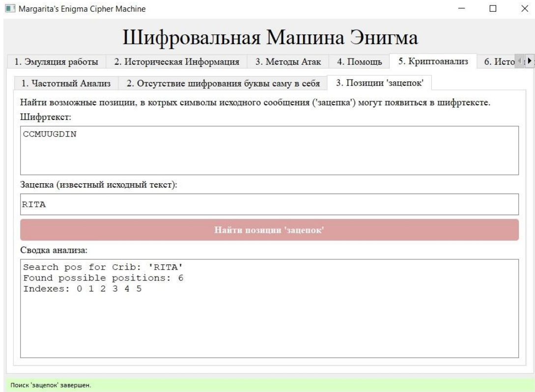
Рис. 17. Вкладка «Криптоанализ» подвкладка «Позиции „зацепок“»
