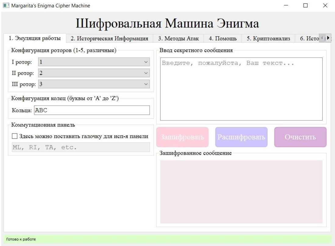
Рис. 5. Главное окно приложения
