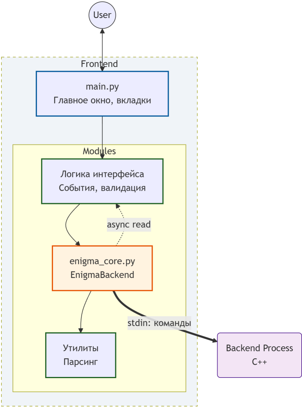
Рис. 2. Схематичное представление архитектуры клиентской части проекта
