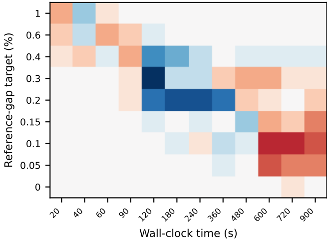
CIPHEUR-online – CIPHEUR-off-EXP
