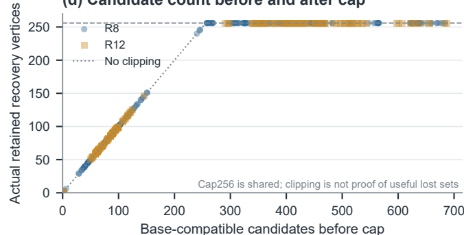
(d) Candidate count before and after cap
