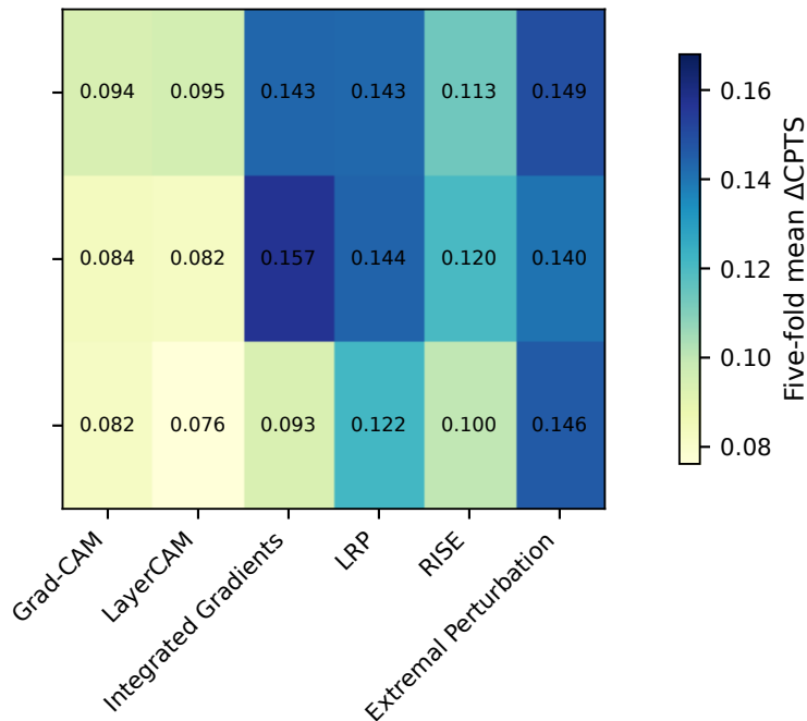
RegNet-X-400MF — 20%
