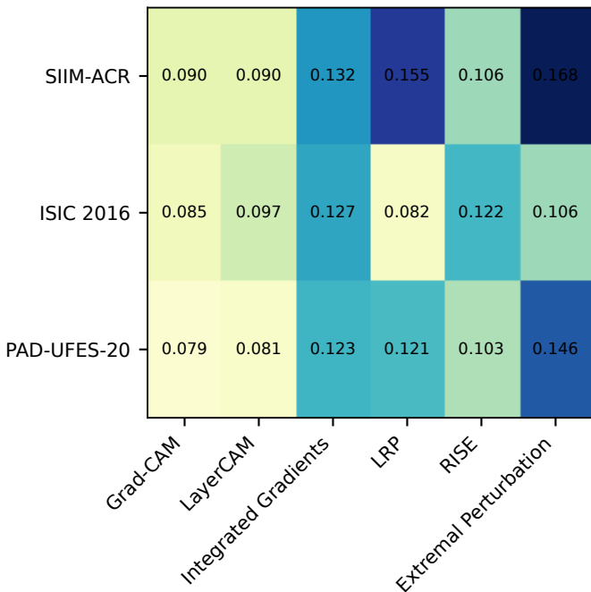
RegNet-X-400MF — 10%
