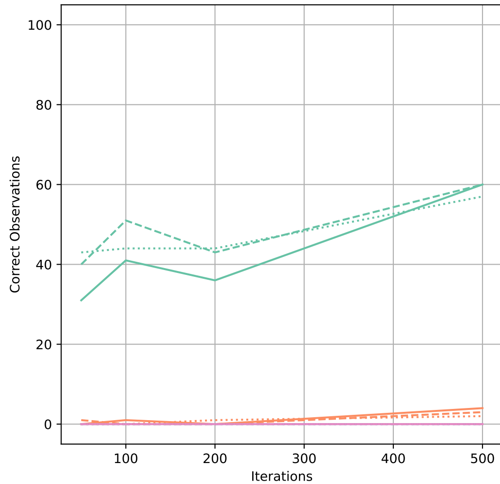
Inlier Deviation: 0.0025
