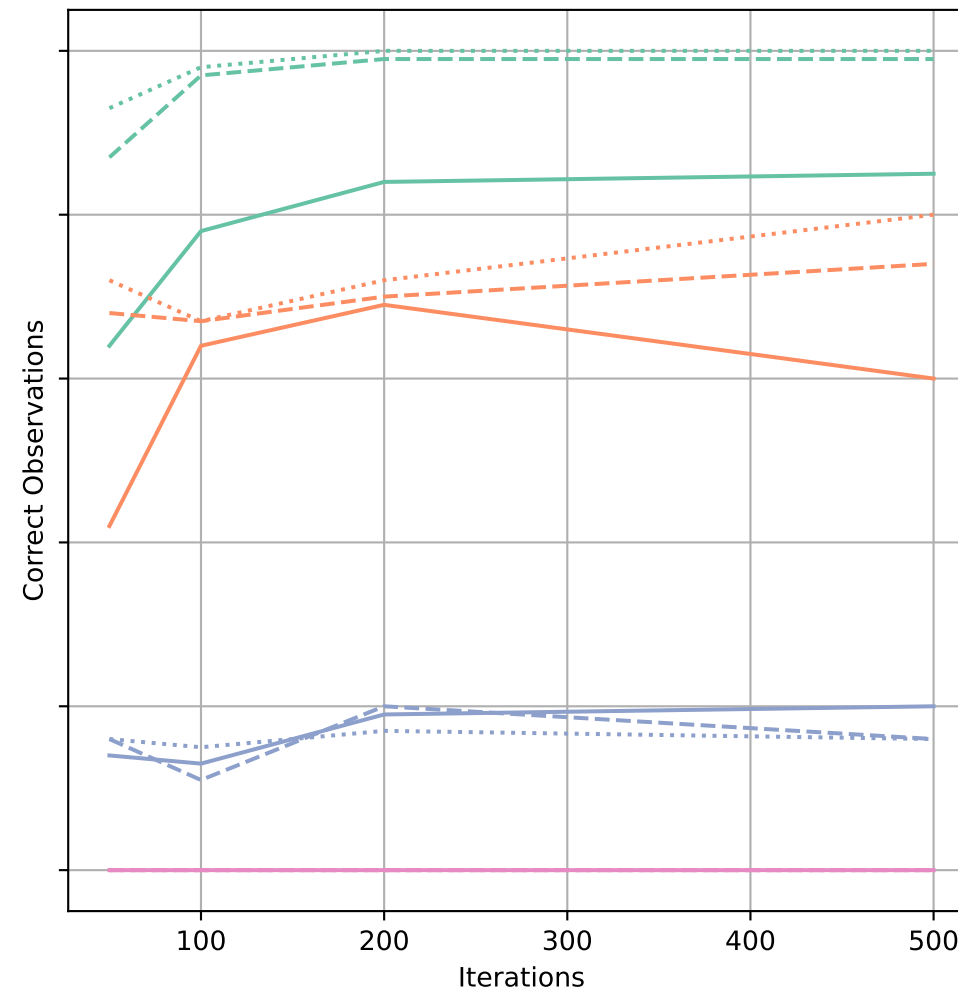
Inlier Deviation: 0.01
