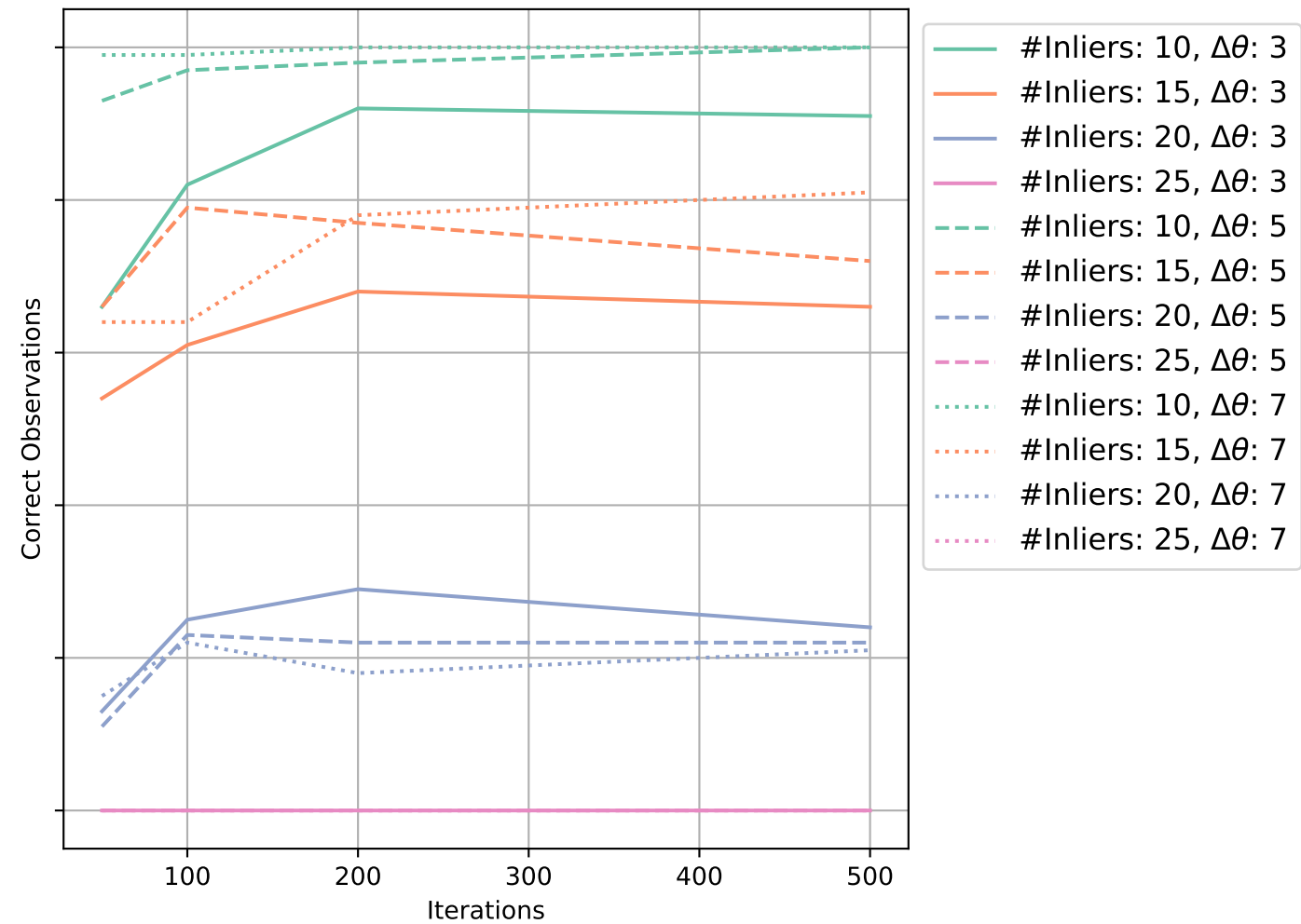
Inlier Deviation: 0.01
