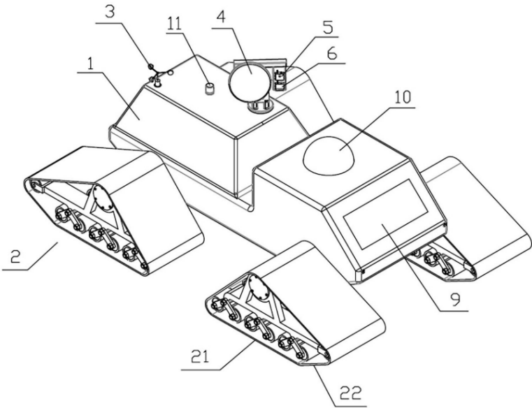
Figura 2.8 Ilustración de robot de inspección con tracción de orugas y sensores climáticos para entornos desérticos.
