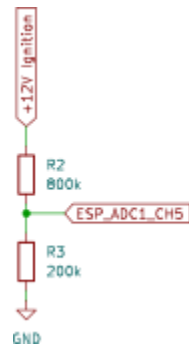
Slika 3.14. Pregled sheme - Djelitelj napona baterije
