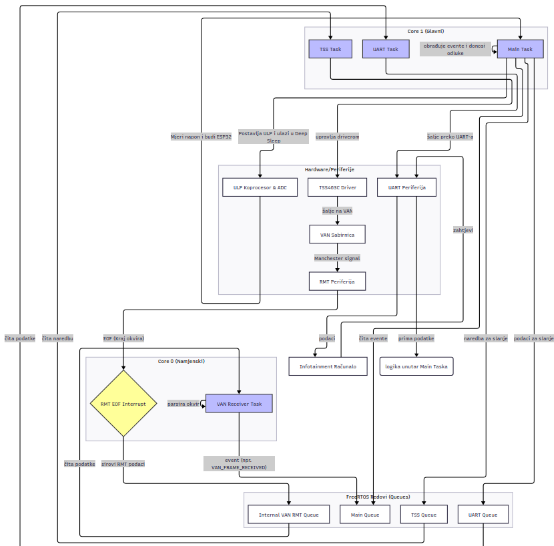
Slika 3.25. Blok dijagram programskog rješenja
