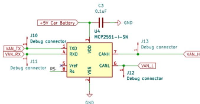
Slika 3.10. Pregled sheme - MCP
