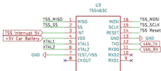
Slika 3.6. Pregled sheme - TSS
