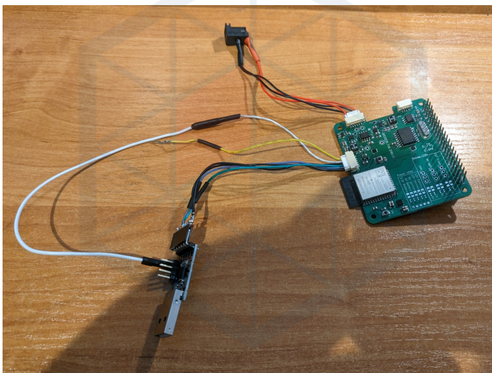
Slika 1: Izgled pristupnog modula sa sklopovljem za programiranje.
