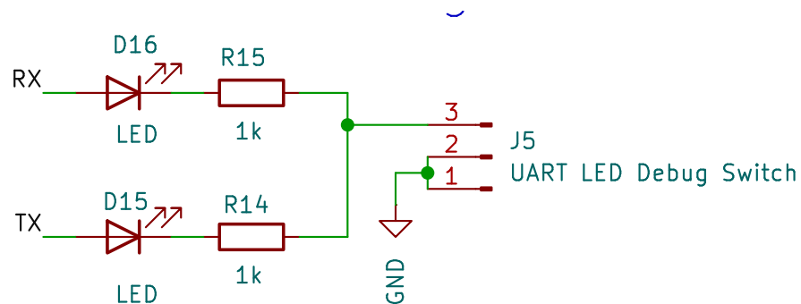
Slika 3.16: Pregled sheme - LE diode za detekciju i otklanjanje žohara na UART sabirnici
