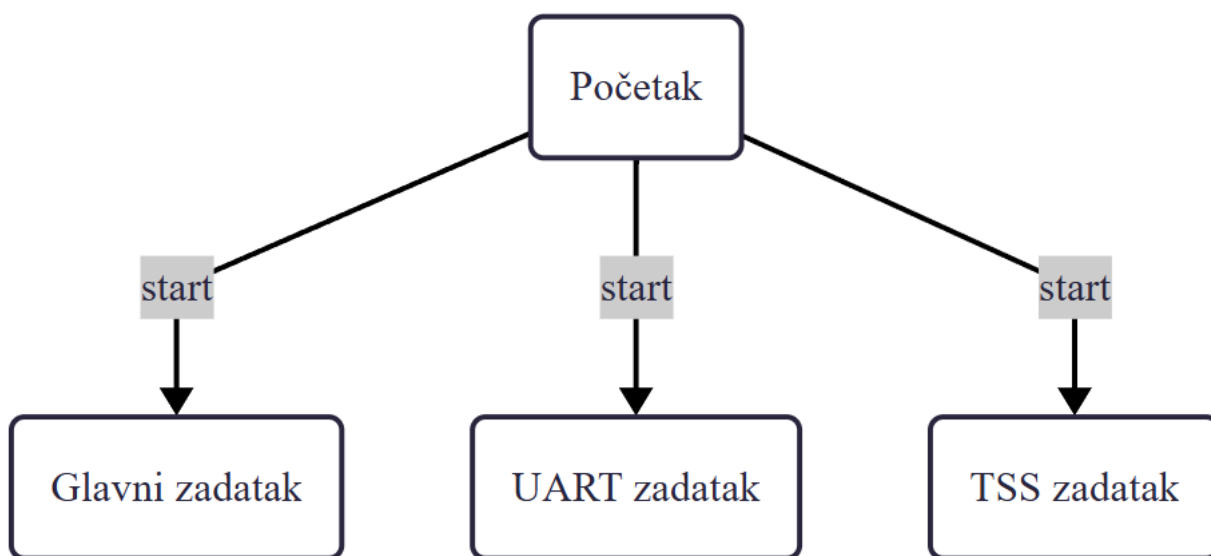
Slika 3.29. Blok dijagram programskog toka - Jezgra 1
