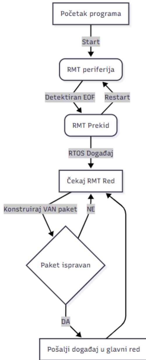
Slika 3.26. Blok dijagram programskog toka - Jezgra 0
