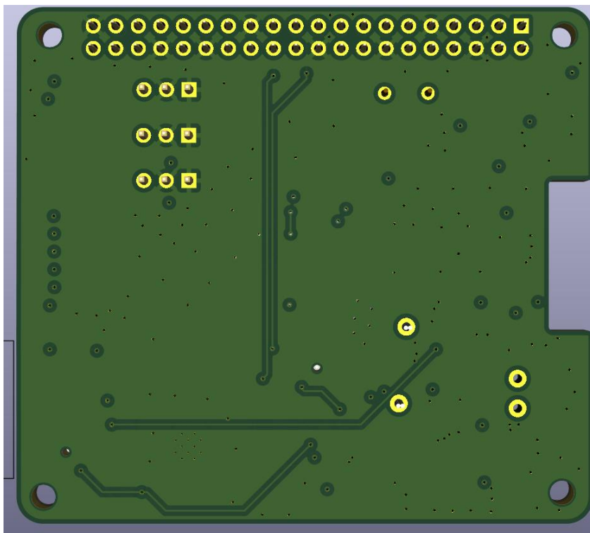
Slika 3.24. Izgled prototipa - PCB zadnja strana.
